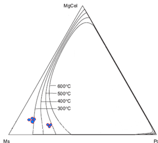
شکل ۱۰. نمودار سولوس میکاهای سفید [۲۹]
