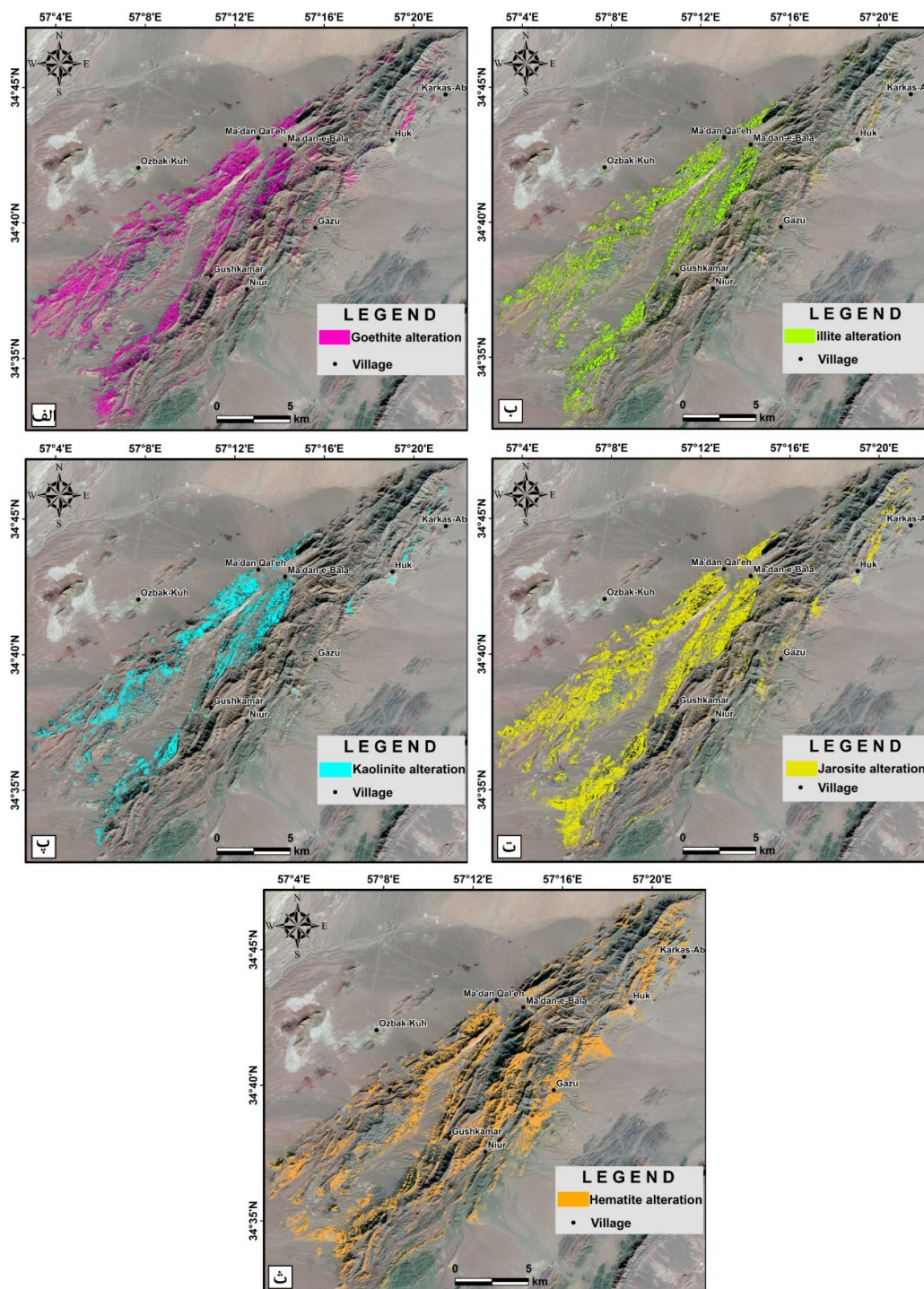
شکل ۲. نقشه دگرسانی‌های استخراج شده از منطقه ازبک‌کوه. الف) دگرسانی گوتیت، ب) دگرسانی ایلیت، پ) دگرسانی کائولینیت، ت) دگرسانی جاروسیت، ث) دگرسانی هماتیت
