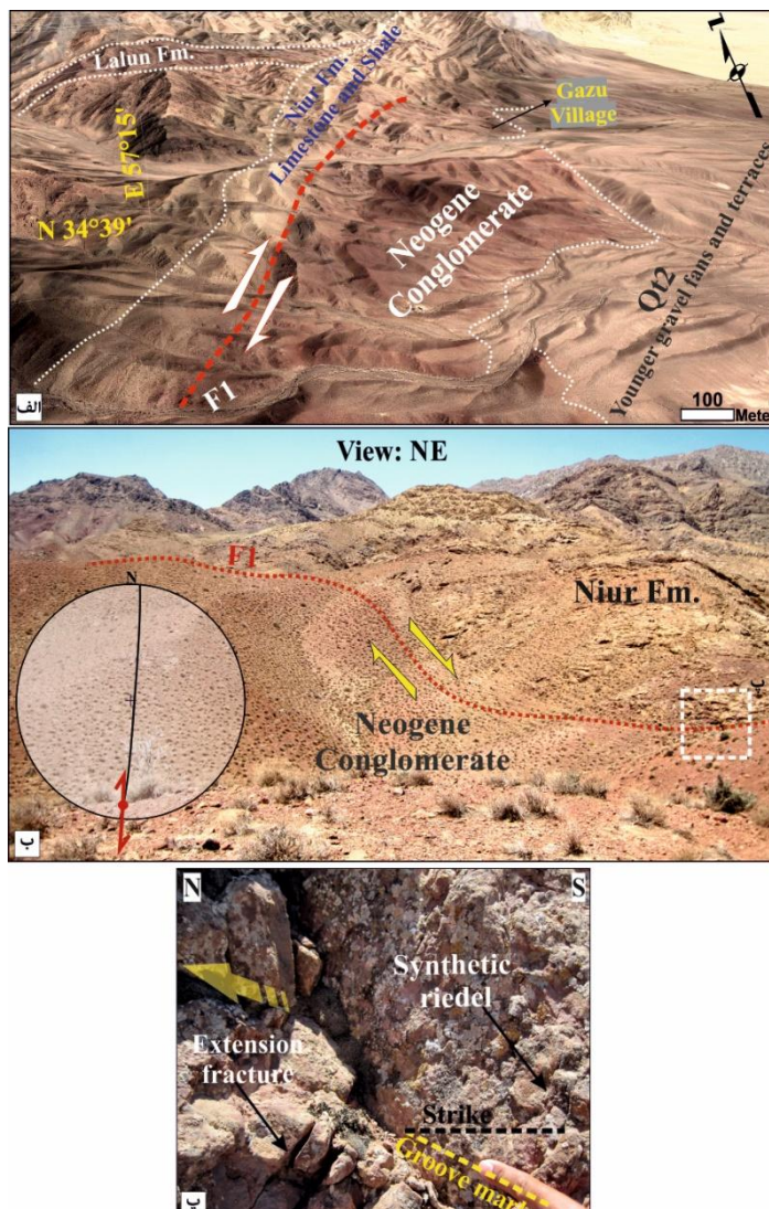
شکل ۳. مشخصات و ویژگی‌های گسل F1. الف) تصویر ماهواره‌ای (Sas planet (Bing map satellite از موقعیت گسل F1، ب) نمایی از گسل F1 در بازدید صحرایی به‌همراه تصویر استریوگرافیک این گسل، پ) شکستگی ریدل و خش خط گسل
