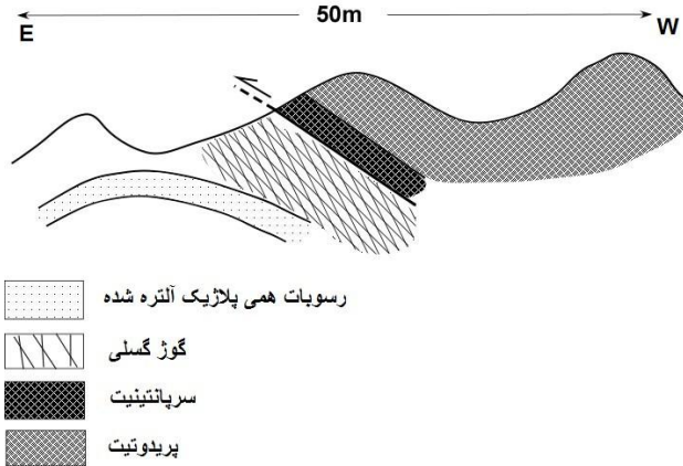
شکل ۲. برش زمین‌شناسی شمال غرب روستای جنگونه که در آن پریدوتیت‌ها با مرز گسله در کنار رسوبات همی پلاژیک قرار گرفته‌اند
