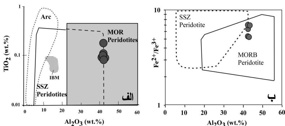
شکل ۱۵ الف. نمودار TiO_2 در مقابل Al_2O_3 کروم اسپینل برای توصیف جای گاه تکتونیکی. داده‌های Izu Bonin Mariana از [۲۴]. ب) نمودار تغییرات Al_2O_3 در مقابل Fe^{2+}/Fe^{3+} در کروم اسپینل. محدوده‌های پریدوتیت‌های بالای زون فرورانش (SSZ) و پشته میان اقیانوسی (MOR) از [۴۸]
