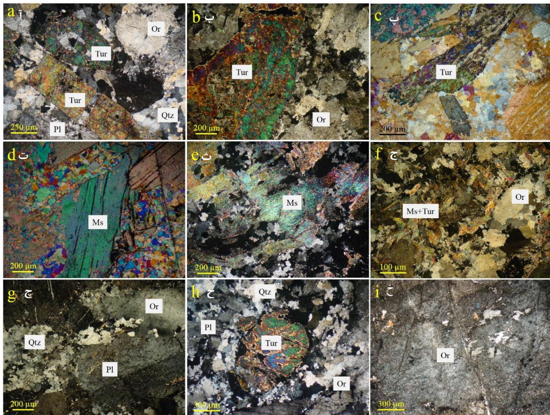
شکل ۴. تصاویر میکروسکوپی (XPL) از پگماتیتهای پهنه بروجرد-نظام‌آباد: (ا) بلورهای خودشکل تورمالین (Tur)، (ب، پ) تورمالین (Tur) و ارتوکلاز (Or) مهم‌ترین کانی‌های تشکیل‌دهنده پگماتیتهای پهنه بروجرد-نظام‌آباد، (ت، ث، ج) بلورهای درشت تاریز موسکوویت (Ms) در پگماتیتهای با میزبان دگرگونی، (چ) ارتوکلاز و پلاژیوکلاز آلبیتی (Pl) درشت بلور در پگماتیتهای با میزبان آذرین، (ح) تورمالین (Tur) نیمه‌شکل‌دار همراه با کوارتز (Qtz) و ارتوکلاز و پلاژیوکلاز، (خ) بلور درشت فلدسپار آلکانل. علایم اختصاری کانی‌ها بر اساس (Whitney & Evans, 2010) است.
