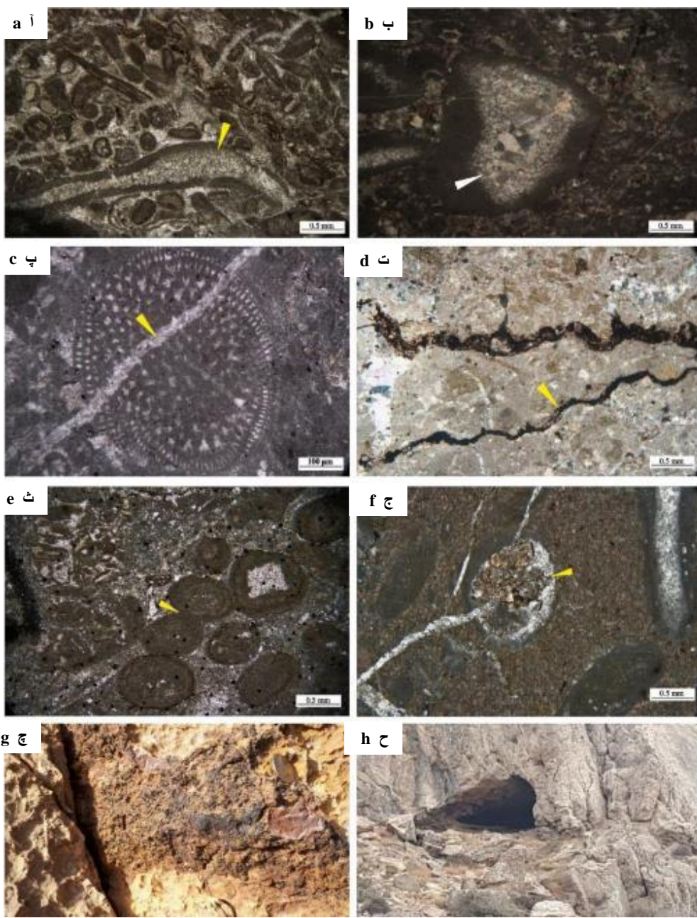
شکل ۹. آ) فرآیند میکریتی شدن در اطراف یک دوکف‌های (فلش زردرنگ) (نمونه ۴Fs)، ب) فرآیند سیمانی شدن از نوع دروزی در درون یک آلوکم (فلش سفید رنگ) (نمونه ۵Fs)، پ) رگه پر شده با سیمان که یک اربیتولینید را قطع کرده است (نمونه ۱۰۰Fs)، ت) استیلولیت‌ها (فلش زردرنگ) (نمونه ۶۶Fs)، ث) تماس خطی دو آنکویید ناشی از فشردگی مکانیکی (فلش زردرنگ) (نمونه ۳Fs)، ج) دولومیتی شدن (فلش زردرنگ) (نمونه ۱۰۰Fs)، چ) آهن‌دار شدن در بخش میانی (نمونه ۸۵Fs) توالی آهکی بررسی شده، ح) تشکیل غار ناشی از فرآیند انحلال و کارستی شدن در ارتفاع ۹۵ متری (دید به سمت جنوب).
