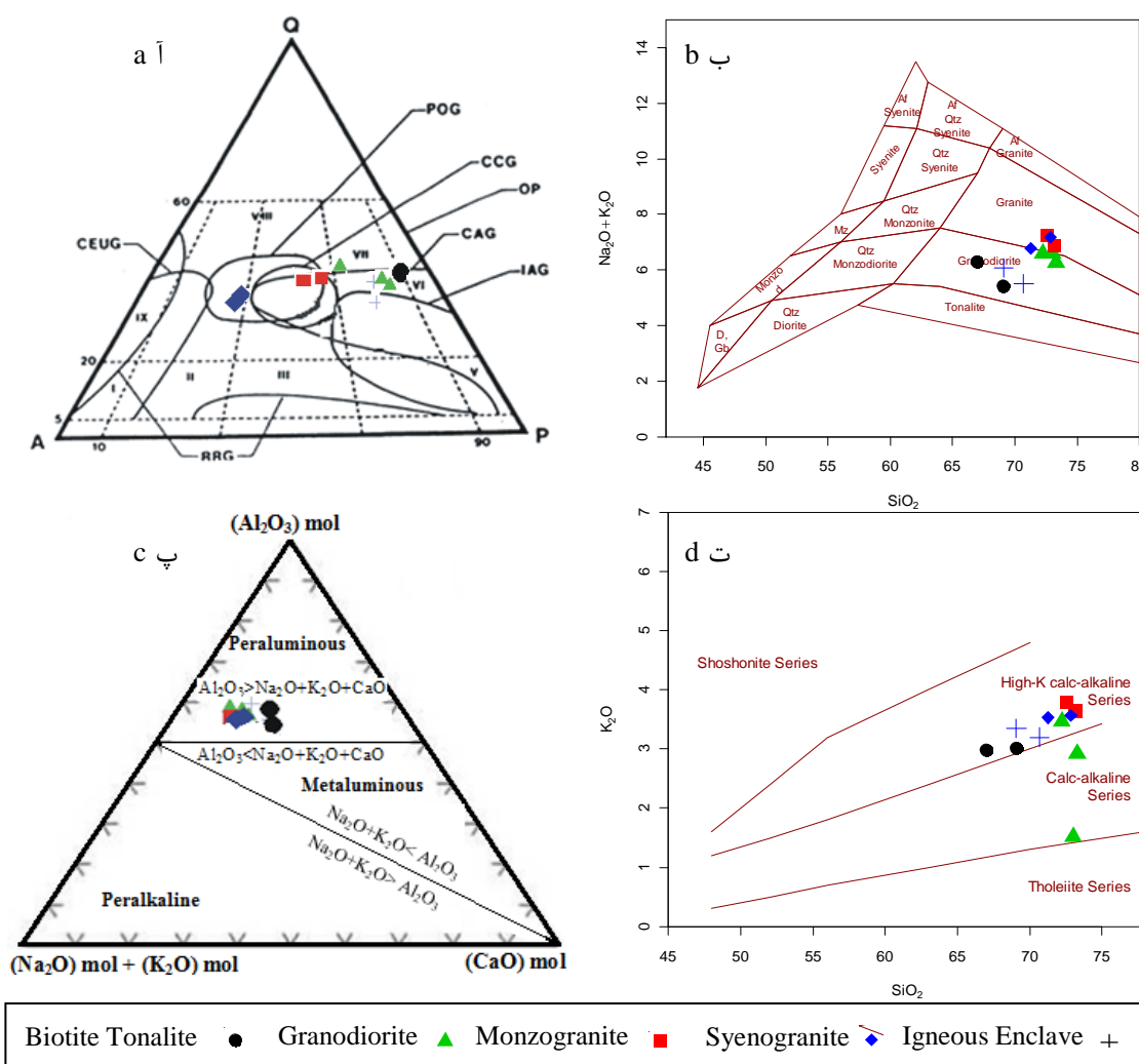
شکل ۶. ا) موقعیت نمونه‌های گرانیتوئید استند در نمودار QAP (Streckeisen, 1976) (IAG: گرانیتوئیدهای جزایر قوسی، CAG: گرانیتوئیدهای حاشیه قاره‌ها، OP: پلاژیوگرانیت‌های اقیانوسی، CCG: گرانیتوئیدهای تصادم قاره‌ای، POG: گرانیتوئیدهای بعد از کوهزایی، CEUG: گرانیتوئیدهای بالاآمدگی اپیروژنیک (خشکی‌زائی)، RRG: گرانیت‌های مرتبط با ریف‌ت، ب) موقعیت نمونه‌های استند در نمودار (Middlemost, 1994)، پ) نمونه‌ها در نمودار (Gill, 2010) در موقعیت پرآلومینوس واقع شده‌اند، ت) نمونه‌ها در نمودار (Peccerillo & Taylor, 1976) بیش‌تر در محدوده کالک‌آلکالین با پتاسیم بالا واقع شده‌اند.
