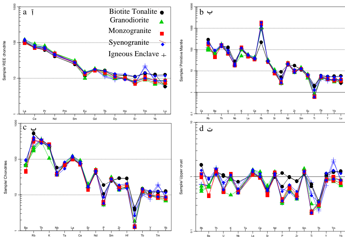
شکل ۹. ا) نمودار عناصر خاکی کمیاب به‌هنجار شده نسبت به کندریت (Nakamura, 1974)، ب) نمودار عناصر خاکی کمیاب به‌هنجار شده نسبت به گوشته اولیه (Sun & Mc Donough, 1989)، پ) نمودار عناصر خاکی کمیاب به‌هنجار شده نسبت به کندریت (Thompson, 1982)، ت) نمودار عناصر خاکی کمیاب به‌هنجار شده نسبت به پوسته بالایی (Taylor & McLennan, 1985).
