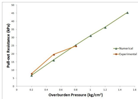
شکل ۲۴- اثر تغییرات فشار سربار اعمالی برای وزن مخصوص خشک 1/6 \text{ gr/cm}^3
