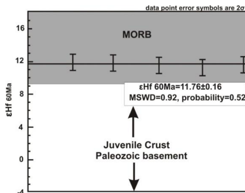
شکل ۱۶. اپسیلون هافنیم اولیه زیرکن‌های گنیس فلسیک که با مقادیر آن در مورب [۵۹] مقایسه شده است.
