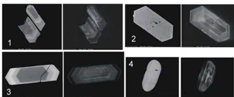
شکل ۱۵. تصاویر BSE ۱ (سمت چپ) و کاتودولومینسانس (سمت راست) زیرکن‌های گنیس فلسیک
