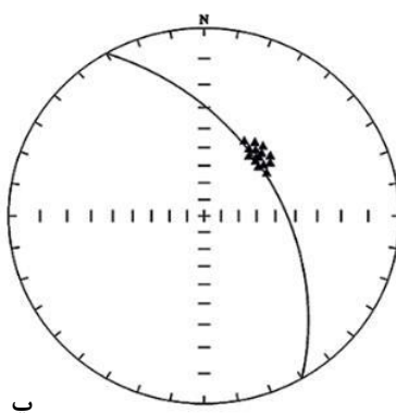
شکل ۶. آ خطواره سایشی رشته‌ای فلدسپات روی صفحه گسل عسگرآباد، در ناحیه عسگرآباد، ب خطواره سایشی رشته‌ای فلدسپات روی صفحه گسل خوی، در ناحیه بدلآباد، پ خط خش‌های سطح گسل در ناحیه بدلآباد - پارچی و عسگرآباد بر صفحه گسل خوی و عسگرآباد
