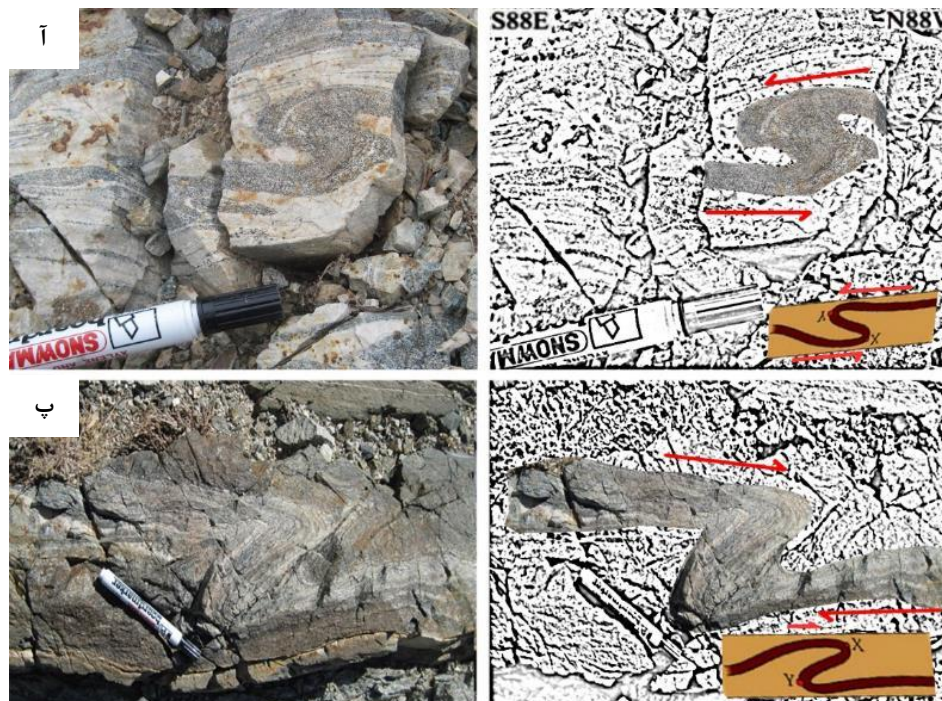
شکل ۱۳. آ) چین‌خوردگی برشی از نوع S شکل در آمفیبولیت گنیسی میلونیتی در روستای بدل‌آباد در منطقه بنگین‌لر در شمال خوی. نوع برش چپ‌گرد است، ب) چین‌خوردگی برشی از نوع Z شکل در گنیسی میلونیتی در روستای بدل‌آباد در منطقه بنگین‌لر در شمال خوی. نوع برش راست‌گرد است.
