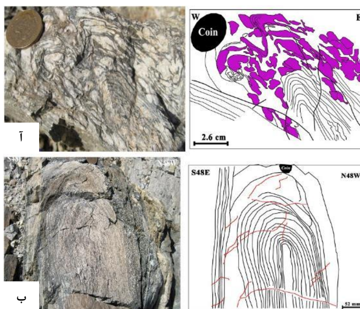
شکل ۱۷. آ) چین‌خوردگی برگوارگی میلوئیتی در آمفیبولیت گنیسی در شمال شرق جاده بدل‌آباد (منطقه قره‌قوشن)- پارچی بالای مرغداری حاج شکر، ب) چین‌خوردگی برگوارگی میلوئیتی در آمفیبولیت گنیسی در منطقه آغاچویلر، شمال بدل‌آباد
