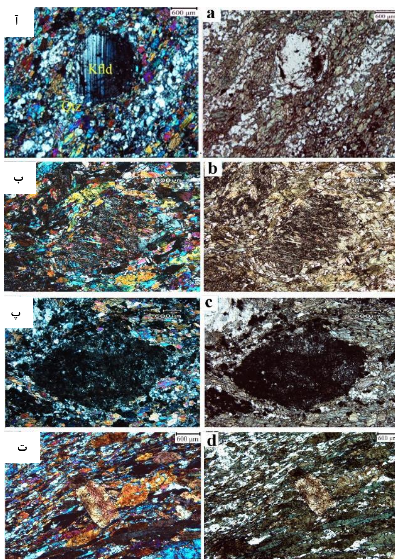
شکل ۱۱. آ) پورفیروبلست فلدسپات پتاسیم‌دار پیش از تکتونیک (D1) در گابروی میلونیتی در ناحیه بدل‌آباد، ب) پورفیروبلست گارنت در آمفیبولیت میلونیتی در شمال خوی در ناحیه بدل‌آباد، پ) پورفیروبلست گارنت در آمفیبولیت میلونیتی در جاده بدل‌آباد- پارچی، سایه‌های واتنشی بدون فیبر در اطراف پورفیروبلست گارنت، ت) پورفیروبلست بیوتیت بعد از تکتونیک (D2) در شیست در شمال غرب خوی در ناحیه بدل‌آباد، نوع حرکت برشی در همه تصاویر راست گرد است. برش موازی با خطوارگی کششی و عمود بر برگوارگی میلونیتی، (a, b, c, d PPL) (A, B, C, D : XPL)
