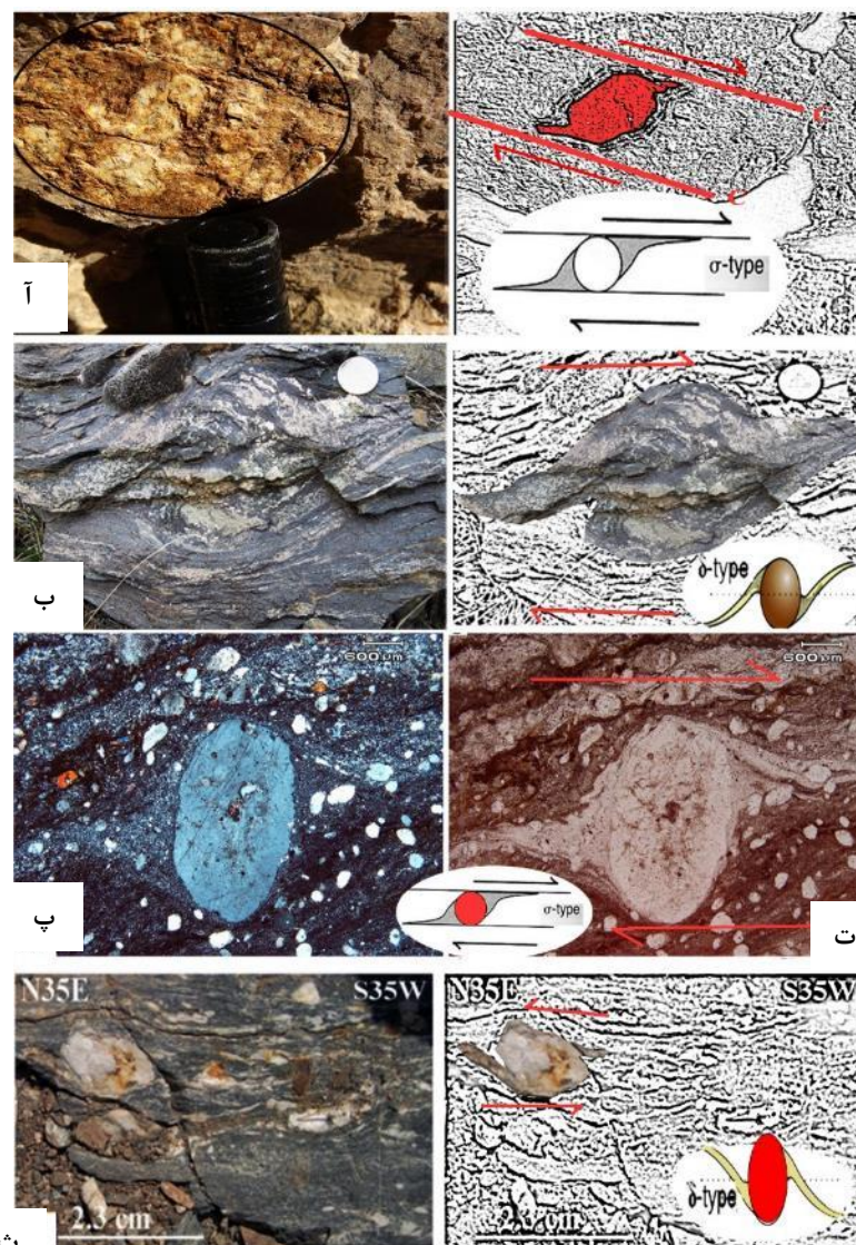
شکل ۱۰. آ) پورفیروکلاست های پوششی از نوع سیگما ( \sigma ) در رخنمون های گرانیتوئیدی منطقه بررسی شده، نوع حرکت برشی راست گرد، ب) پورفیروکلاست های پوششی از نوع دلتا ( \delta ) در رخنمون های متابازیتی منطقه بررسی شده، نوع حرکت برشی راست گرد، پ) گابرو میلونیتی با پورفیروکلاست های پوششی سیگما ( \sigma ) با جنس فلدسپار پتاسیم دار، برگوارگی با روندی از سمت راست بالا به طرف سمت چپ پایین مشاهده می شود. نوع حرکت برشی راست گرد، برش موازی با خطوارگی کششی و عمود بر برگوارگی میلونیتی (C : CPL, D: PPL, ث) گرانیتوئید میلونیتی با پورفیروکلاست های پوششی نوع دلتا ( \delta ) از جنس فلدسپار پتاسیم در منطقه بنگلین لر شمال بدل آباد، نوع حرکت برشی چپ گرد
