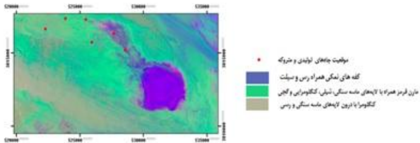
شکل ۱۵. تصویر ترکیب سه باند اولیه روش MNF
