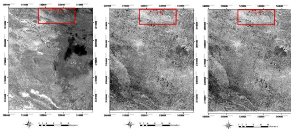
شکل ۸. چپ) تصویر نسبت باندهای (7+9)/8 که در آن مناطق روشن نشان‌دهنده کربنات است، وسط) تصویر تحلیل مؤلفه اصلی با مقدار مؤلفه اصلی باند ۵ که در آن مناطق روشن نشان‌گر کربنات است، راست) تصویر کم‌ترین مربعات با باندهای مدل ۷ و ۹ که در آن مناطق روشن بسترهای کربناته است.
