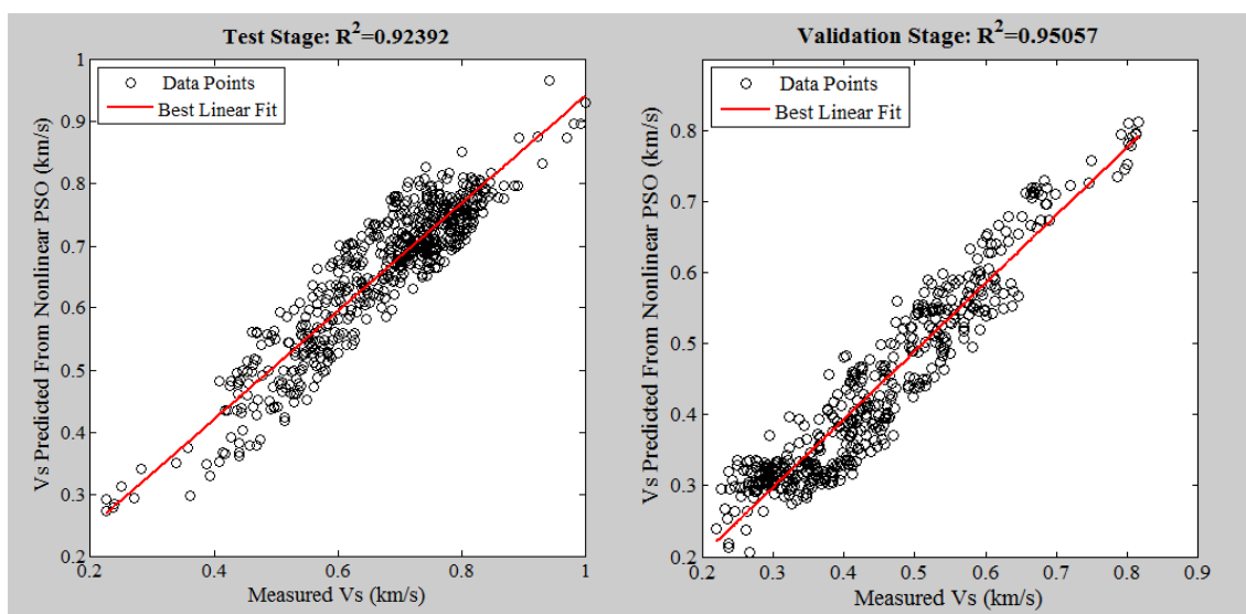
شکل ۶. مقادیر ضریب هم بستگی بین Vs حاصل از مدل غیرخطی PSO و Vs اندازه گیری شده از DSI در داده های تست و
