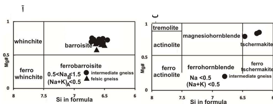
شکل ۷. مطابق نمودارهای تقسیم‌بندی آمفیبول [۲۷]، آمفیبول گنیس‌های فلسیک از (آ) نوع بارونیزیت (ب) و انواع حدواسط از نوع بارونیزیت و ندرتاً چرماکیت و فروهورنبلند هستند.
