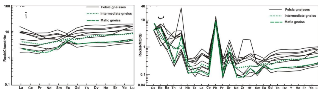
شکل ۱۲. آ) در نمودار سنجدیده شده نسبت به کندریت [۴۹]، الگوی عناصر نادر خاکی گنیس‌های مجموعه دگرگونی سلطان‌آباد دارای شیب مثبت هستند. ب) غنی‌شدگی از عناصر U, Cs, Sr و Rb و تهی‌شدگی از Ta و Nb در نمودار سنجدیده شده نسبت به مورب [۵۱]، نمایان است.
