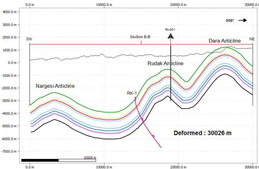
شکل ۲۰. طول نهایی مقطع B-B' در حالت چین خورده و وضعیت چین خوردگی قبل از بازگرداندن لایه‌ها به مرحله قبل از دگرشکلی
