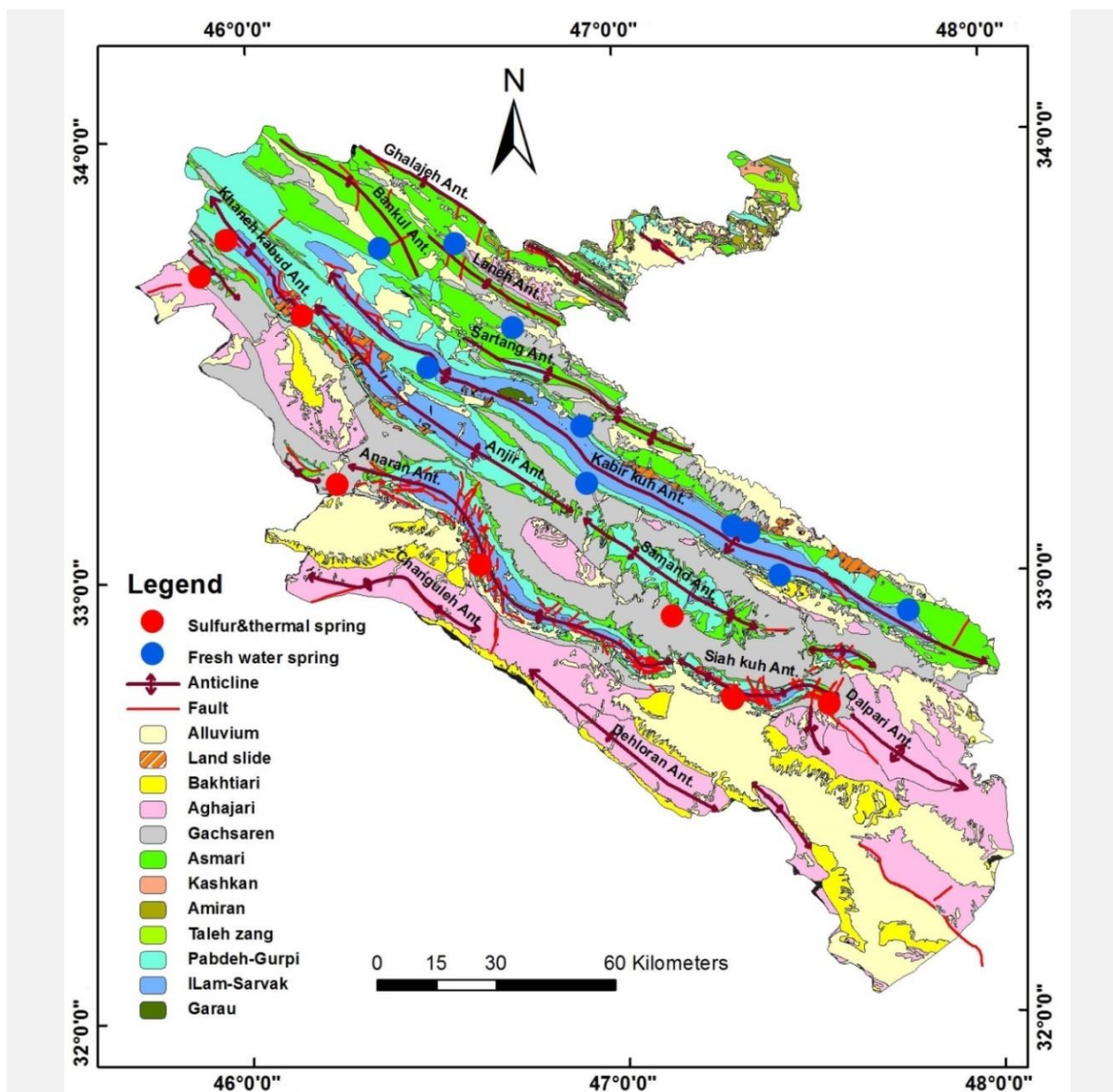
شکل ۲. نقشه زمین‌شناسی و تکتونیک استان ایلام اقتباس از نقشه‌های زمین‌شناسی دهلران (Llewellyn, 1973) و ایلام-کوهدهشت (Llewellyn, 1974)
