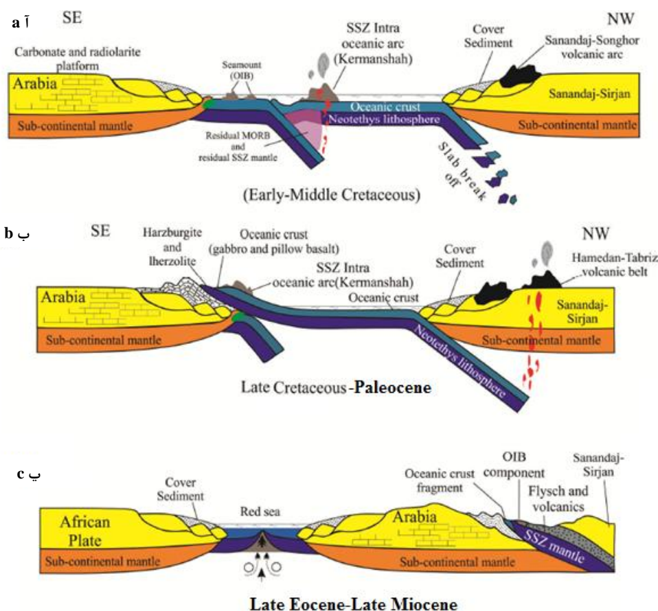
شکل ۱۰. مدل شماتیک (بدون مقیاس) و پیشنهادی برای تکامل و نحوه تشکیل افیولیت کرمانشاه در منطقه کامیاران (Moradpour, 2017). با اندکی تغییر
