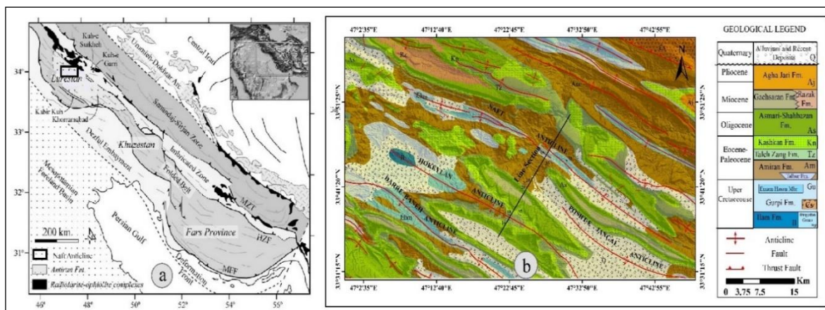
شکل ۱- (a) نقشه جایگاه ساختاری و زیرپهنه های تکتونیکی کمربند چین خورده رانده زاگرس در جنوب باختر ایران که موقعیت منطقه مورد مطالعه در کمربند چین خورده-رانده زاگرس با مستطیل سیاه رنگ مشخص شده است (Homke et al., 2004). (b) نقشه زمین‌شناسی منطقه مورد مطالعه در پهنه لرستان، موقعیت نیمرخ ساختاری با خطوط سیاه رنگ مشخص شده است.
