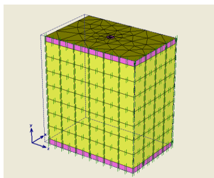
شکل ۷- شرایط مرزی مدل ساخته شده
