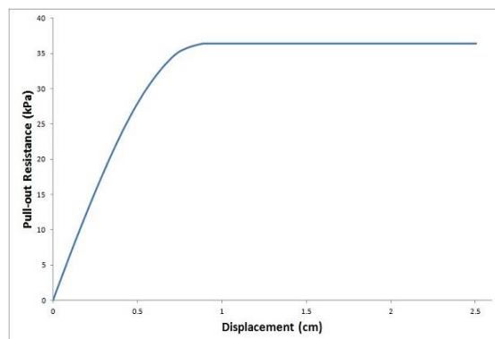
شکل ۲۰- تغییرات مقاومت در برابر تغییرمکان میخ B5 Fig. 20. Changes in strength to nail displacement B5
