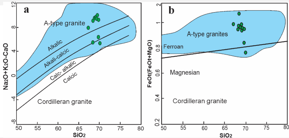
شکل ۹- نمودار (a) \text{Na}_2\text{O}+\text{K}_2\text{O}-\text{CaO} در مقابل \text{SiO}_2 (Frost et al., 2001). نمودار (b) \text{FeO}^t/(\text{FeO}^t + \text{MgO}) نسبت در مقابل \text{SiO}_2 (Frost et al., 2001). محدوده آبی رنگ معرف دامنه ترکیب شیمیایی گرانیت‌های نوع A است (Vander Auwera et al., 2003).
