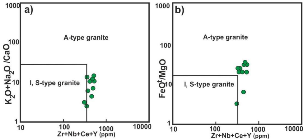
شکل ۸- نمودارهای متمایز کننده گرانیت‌های نوع A از گرانیت‌های نوع I و S (Whalen et al., 1987). نمودار (a) (\text{Na}_2\text{O}+\text{K}_2\text{O})/\text{CaO} در برابر \text{Zr}+\text{Nb}+\text{Ce}+\text{Y} (ppm) نمودار (b) \text{FeO}^t/\text{MgO} در برابر \text{Zr}+\text{Nb}+\text{Ce}+\text{Y} (ppm) نمودار (b) (\text{Na}_2\text{O}+\text{K}_2\text{O})/\text{CaO} نسبت برابر نسبت A-type= Anorogenic type, I and S type= Igneous and Sedimentary types
