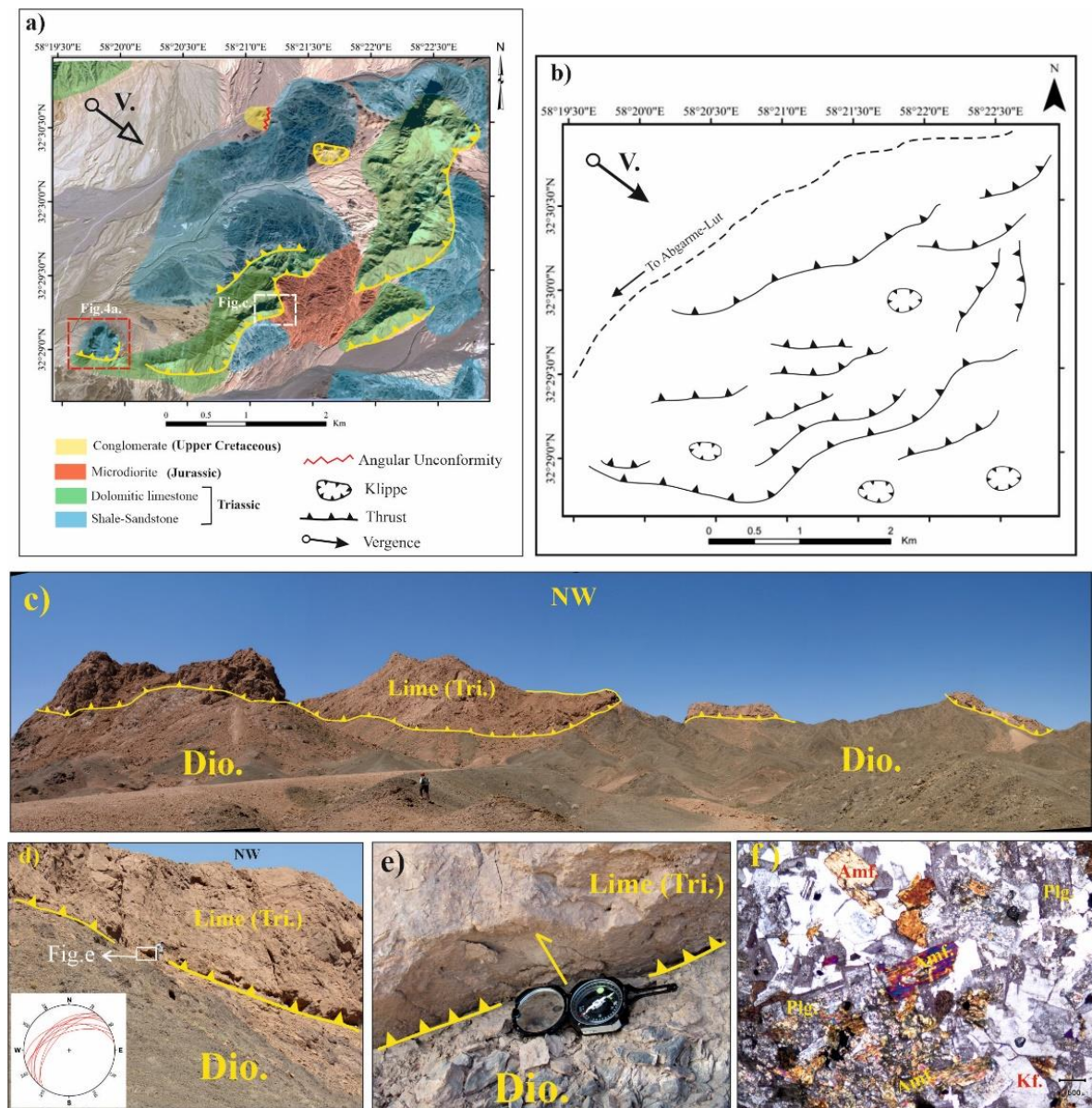
شکل ۳- (a) ارتباط بین واحدهای زمین‌شناسی مختلف با صفحات راندگی در منطقه سه‌چنگی. V.: جهت انتقال زمین‌ساختی. (b) نقشه ساختاری از راندگی‌های شکل a. (c) تصویر پانوراما از راندگی آهک‌های تریاس (Tri.) بر روی میکرودیوریت‌های ژوراسیک (Dio.). (d) کنتاکت گسلش راندگی بین آهک و میکرودیوریت. کادر روی تصویر در شکل e بزرگنمایی شده است. (e) صفحه گسلش راندگی با شیب به سمت شمال غرب. (f) مقطع نازک میکروسکوپی از میکرودیوریت منطقه سه‌چنگی. بافت میکروگرانولار شامل کانی‌های فلدسپار (Kf)، پلاژیوکلاز (Plg.) و آمفیبول (Amf.). نورپلاریزه با بزرگنمایی ۴۰ برابر.
