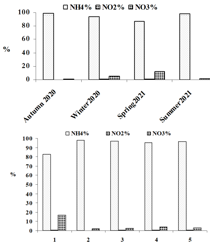
شکل ۴- تغییرات درصد فرم‌های مختلف نیتروژن معدنی در فصول و ایستگاه‌های مختلف حوضه آبریز سد زاوه-سنندج (۱۴۰۰-۱۳۹۹) Fig. 4. Changes of different forms of inorganic nitrogen in different seasons and stations in the catchment area of the Zhaveh Dam of Sanandaj (2020-2021)
