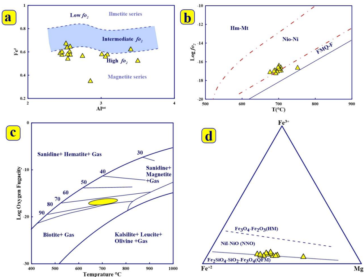
شکل ۸- موقعیت بیوتیت‌های موجود در گرانودیوریت‌های توده گودحوض در نمودارهای مختلف تعیین‌گر زندگی اکسیژن. (a) نمودار عدد آهن (Fe#) در مقابل آلومینیم کل ( Al^{tot} ) (Anderson et al., 2008). (b, c) نمودار \log fO_2 -T (Wones and Eguster, 1965; Wones, 1980). (d) نمودار سه تایی Fe^{2+} - Fe^{3+} -Mg (Wones and Eguster, 1965).
