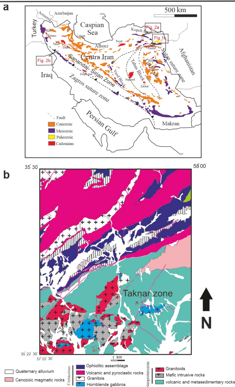
شکل 1- (a) نقشه ساده زمین‌شناسی ایران که در آن توزیع سنگ‌های آذرین سنوزوئیک، مزوزوئیک، پالئوزوئیک و کادومیان نشان داده شده است. موقعیت محدوده‌های مورد مطالعه با مستطیل مشخص شده‌اند. (b) نقشه زمین‌شناسی منطقه کبودان (Mazhari et al., 2020). Fig. 1. a) A simplified geological map delineating the distribution of Cenozoic, Mesozoic, Palaeozoic, and Cadomian igneous formations in Iran. The rectangular outline denotes the location of the studied areas. b) Geological map of the Kaboodan area (Mazhari et al., 2020).
