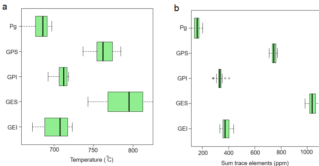
شکل ۸-ا) مقایسه دمای محاسبه شده با روش Titan Q بلورهای کوارتز در انواع گرانیتوئیدهای مورد مطالعه. (b) تفاوت مجموع عناصر کیمیايي در انواع گرانیتوئیدها. : گرانیتوئیدهای نوع S در منطقه کبودان؛ GPI: گرانیتوئیدهای نوع I در منطقه کبودان؛ GES: گرانیتوئیدهای نوع S در مجموعه نفوذی بانه؛ GEI: گرانیتوئیدهای نوع I در مجموعه نفوذی بانه؛ Pg: پلاژیوگرانیت‌های سبزوار.
