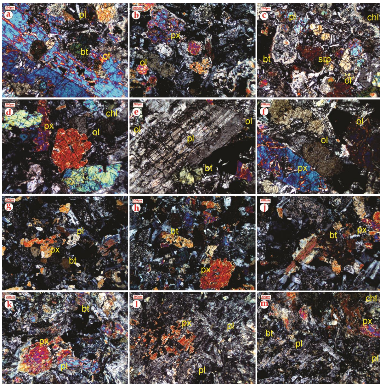
شکل ۴- تصاویر میکروسکوپی سنگ‌های آذرین مورد مطالعه. کانی‌های پلاژیوکلاز (Pl)، پیروکسن (Px) و الیوین (Ol) کانی‌های اصلی در این سنگ‌ها می‌باشند. کانی‌های کلینوپیکروکسن معمولاً به کانی‌های ثانویه مانند مگنتیت، بیوتیت (Bt) و کلریت (Chl) تبدیل شده‌اند. Chl = کلریت، Opq = کانی‌های مات، Pl = پلاژیوکلاز، Px = پیروکسن، Ol = الیوین، Srp = سرپانتین. علائم اختصاری کانی‌ها برگرفته شده از وایتنی و اوانس (Whitney and Evans, 2010) می‌باشد.
