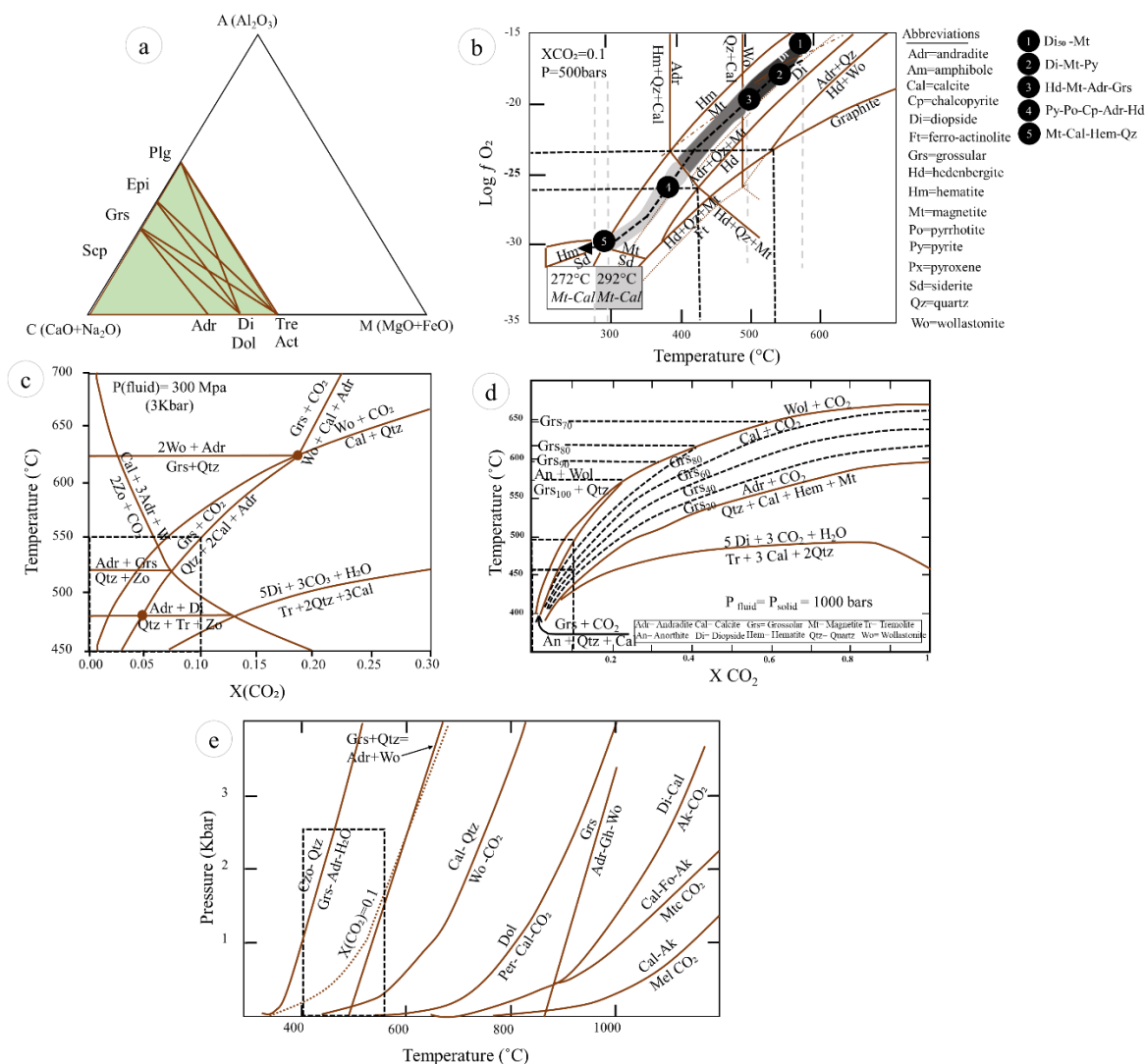
شکل ۷- (a) نمایش مجموعه کانی‌های پهنه‌های اسکارنی تپه‌قرمز و روابط بین آن‌ها در نمودار ACM (Sengupta et al., 1989)، که در آن \text{CO}_2 ، \text{H}_2\text{O} ، \text{Qtz} به صورت فاز اضافی در نظر گرفته شده است، (b) نمودار اصلاح شده \text{T-Log}f\text{O}_2 که محدوده پایداری کانی‌های کالک سیلیکاته اسکارنی، اکسیدها، سولفیدها و کانی‌های کربناته را نشان می‌دهد، پیشنهادی اینودی (Einaudi, 1982a) که از اویمان (Oyman, 2010)، اقتباس شده است، (c) نمودار دما در برابر \text{XCO}_2 در فشار سیال ۳ کیلو بار برای سیستم Si-Al-Mg-Ca-C-O-H پیشنهادی پرکینز و همکاران (Perkins et al., 1986)، که از چاودهوری و لنتز (Chowdhury and Lentz, 2011) اقتباس شده است، (d) نمودار \text{T-XCO}_2 در \text{P}_{\text{fluid}} = 1000 \text{ bar} (اقتباس از سوئنی (Sweeney, 1980)). \text{Grs}_{100} ، گارنت کلسیم-آلمینیوم دار خالص (گرو سولار)، \text{Adr} ، آندرادیت خالص گارنت کلسیم-آهن دار (آندرادیت)، و \text{Grs}_{20} - \text{Grs}_{80} محلول جامد آندرادیت-گرو سولار است، (e) نمودار
