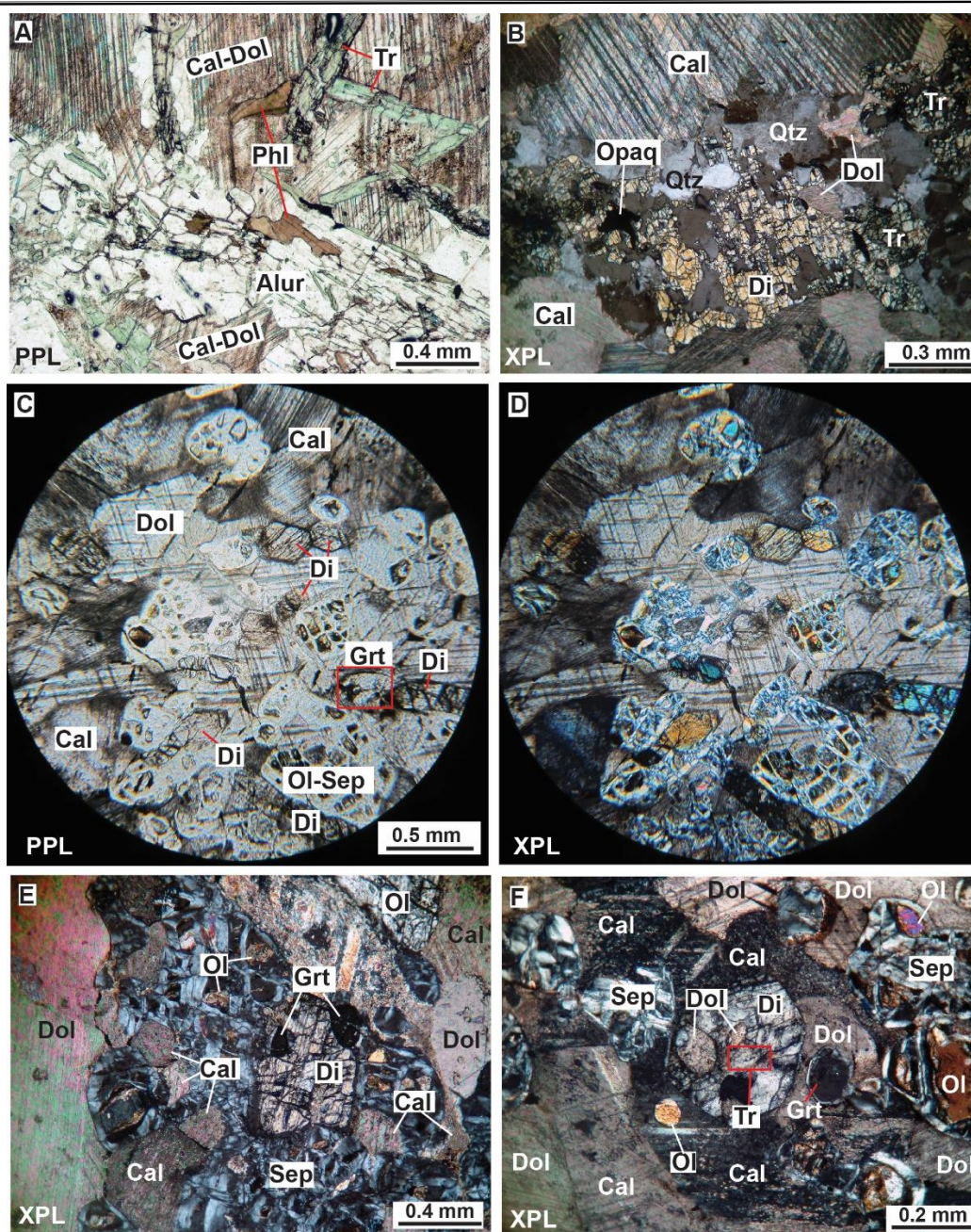
شکل ۳- تصاویر میکروسکوپی از سنگ‌های مرم‌های دولومیتی مجموعه دگرگونی قوری. a و b) رخداد گردهمایی کانیایی ترمولیت + فلوگوپیت + کلسیت + دولومیت + آلورژیت (نوعی میکای سفید) و دیوپسید + ترمولیت + دولومیت + کلسیت + کانی کدر در سنگ‌های با درجه دگرگونی ضعیف تا متوسط در طول مرحله رشد M1 (به شکل ۶ مراجعه شود). c و d) رخداد گردهمایی کانیایی الیوین + گارنت + دیوپسید + کلسیت + دولومیت در سنگ‌های با درجه دگرگونی قوی در طول مرحله رشد M1. الیوین‌ها در مراحل بعدی دگرگونی سرپانتینی (آنتی‌گوریت) شده‌اند. e و f) رخداد گردهمایی کانیایی الیوین + گارنت + دیوپسید + کلسیت + دولومیت در سنگ‌های با درجه دگرگونی قوی در طول دگرگونی از مرحله M1 به سمت مرحله M2. الیوین‌ها در مراحل بعدی دگرگونی سرپانتینی شده‌اند. همچنین بقایای ترمولیت با درجه دگرگونی متوسط در داخل دیوپسیدها به دام افتاده است. این گردهمایی‌های کانیایی مراحل انتهایی رشد دگرگونی M1 را نشان
