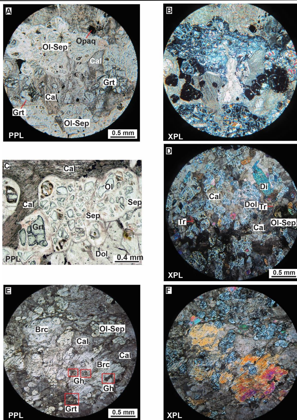
شکل ۴- تصاویر میکروسکوپی از سنگ‌های مرمر دولومیتی مجموعه دگرگونی قوری. a و b) رخداد گردهمایی کانیایی الیون + گارنت + دیوپسید + کلسیت + دولومیت در سنگ‌های با درجه دگرگونی قوی در طول دگرگونی M1 به سمت M2 که در مراحل بعدی دگرگونی (انتهای M2)، الیون به سرپانتین (آنتی‌گوریت) و گارنت به سرپسیت و کلریت (پنینیتی شدن) تبدیل شده‌اند. c و d) رخداد گردهمایی کانیایی الیون + دیوپسید + کلسیت + دولومیت + کانی کدر در سنگ‌های با درجه دگرگونی قوی در طول دگرگونی M2 (به شکل ۶ مراجعه شود). الیون‌ها در مراحل بعدی دگرگونی الیون، سرپانتینی (آنتی‌گوریت) شده‌اند و بلورهای
