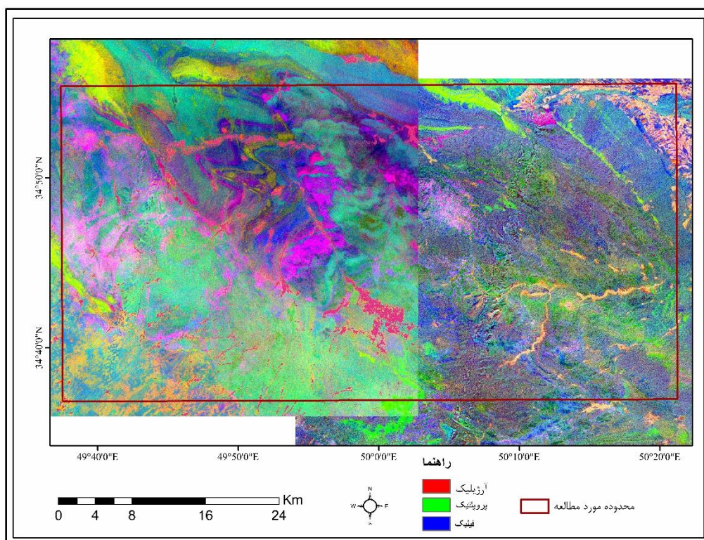
شکل ۱۶- نتیجه نهایی پردازش به روش آنالیز مولفه های اصلی انتخابی. محدوده هایی با گام صورتی کمرنگ تا قرمز نمایان گر دگرسانی آرژیلیک و محدوده های سبز و زرد نشان دهنده دگرسانی پروپلیتیک و مناطق با رنگ آبی تا بنفش دگرسانی فیلیک می باشند.
