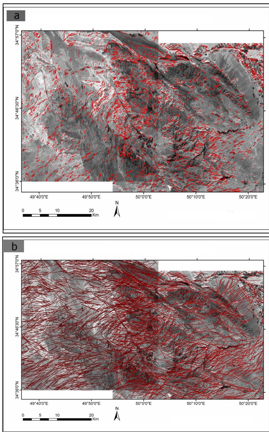
شکل ۶- (a) استخراج خطواره‌ها با پارامترهای خطواره کوتاه. (b) استخراج خطواره‌ها با پارامترهای خطواره‌های بلند برای همان تصویر
