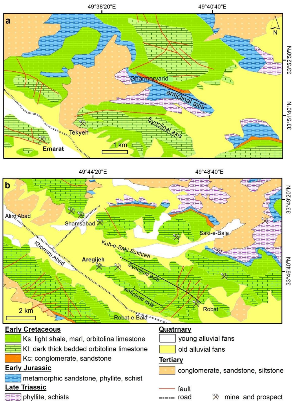
ش‌ک‌ل ۲- ن‌ق‌شه ز‌م‌ی‌ن‌ش‌ن‌اس‌ی س‌اده ش‌ده ( بر‌اس‌اس ن‌ق‌شه ی‌ک‌ص‌د ه‌زار و‌ر‌چه، ) (ا منطقه اره‌گی‌جه، ب) م‌عدن ع‌مارت (Vaezi and Kholghi, 2007).
