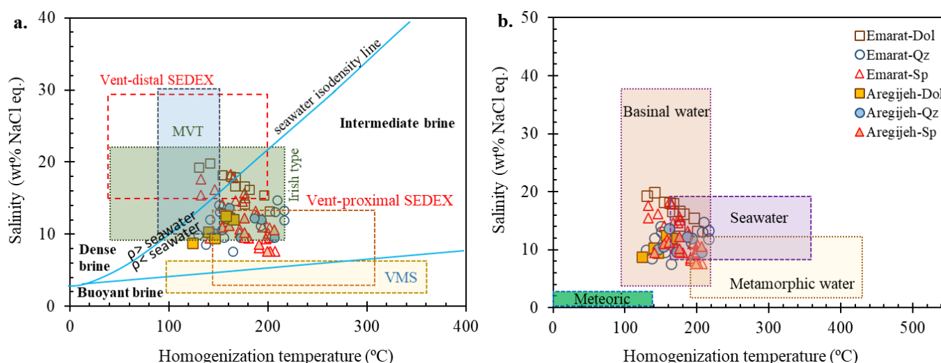
شکل ۱۱- (a) نمودار دمای همگن‌شدگی در برابر شوری (معادل درصد نمک طعام) که نشان می‌دهد میانبارهای سیال در محدوده کانسارهای نوع ایرلندی قرار گرفته‌اند (Wilkinson et al., 2009; compiled by Rajabi et al., 2015 and Yarmohammadi et al., 2016). (b) نمودار محدوده‌های آب مختلف پیشنهادی از کسler (Kessler, 2005).
