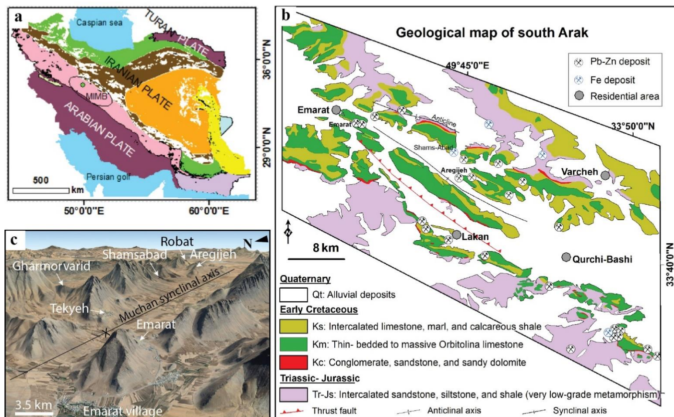
شکل ۱. ا) نقشه زمین‌شناسی- ساختاری ایران شامل موقعیت کمربند فلززایی ملایر-اصفهان (MIMB) و کانسار اره‌گیجه (Aghanabati, 2013). ب) کانسارهای سرب- روی و آهن بر روی نقشه ساده زمین‌شناسی منطقه جنوب اراک نشان داده شده است (Vaezi and Kholghi, 2007). منطقه معدنی اره‌گیجه در جنوب خاوری معادن عمارت و شمس‌آباد قرار دارد، ج) موقعیت منطقه مورد مطالعه بر روی تصویر گوگل ارث، زمینه تصویر در سامانه جغرافیایی WGS84 است.
