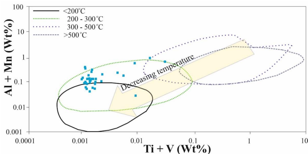
شکل ۷- تعیین دمای تشکیل مگنتیت‌های میدوک با استفاده از شیمی کانی مگنتیت بر روی نمودار \text{Al}+\text{Mn} در برابر \text{Ti}+\text{V} (Deditius et al., 2018) Fig. 7. \text{Al}+\text{Mn} vs. \text{Ti}+\text{V} diagram used to estimate crystallization temperature of magnetite (Deditius et al., 2018)
