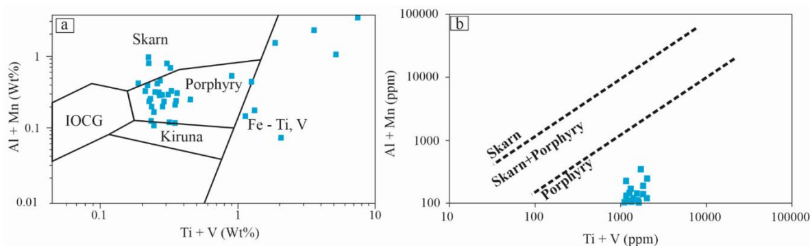
شکل ۶- a) موقعیت نمونه‌های مگنتیت کانسار میدوک بر روی نمودار Al + Mn در برابر Ti + V (Nadoll et al., 2015)؛ b) وضعیت قرارگیری نمونه‌های شیمی کانی مگنتیت کانسار میدوک Al + Mn در برابر Ti + V (Nadoll et al., 2014)
