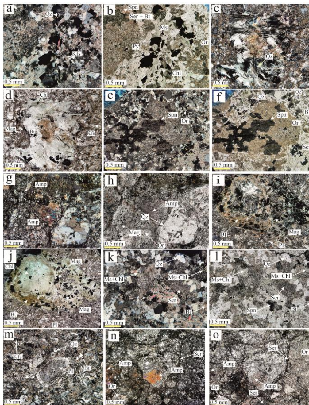
شکل ۲- تصاویر میکروسکوپی از کانی‌های سیلیکاتی گرانیت‌های کانسار میدوک: (a و b) بلورهای کوارتز با ساختار پر مانند، دگرسانی ارتوکلاز به سریسیت، دگرسانی بیوتیت به کلریت، کانی‌های فرعی و بدون شکل اسفن و پیریت و بلورهای شکل‌دار مگنتیت (شاخص زون پتاسیک در سنگ گرانیت) (a: نور XPL و b: نور PPL)، (c و d) بلورهای کوارتز با ساختار پر مانند، دگرسانی بیوتیت به کلریت، بلورهای ریز نیمه شکل‌دار مگنتیت، دگرسانی بالا فلدسپار پتاسیم به سریسیت (معرف زون پتاسیک در سنگ گرانیت) (c: نور XPL و d: نور PPL)، (e و f) بلورهای ریز بدون شکل کوارتز، بلورهای خیلی کم بیوتیت، دگرسانی ارتوکلاز به سریسیت، کانی فرعی اسفن با برجستگی تقریباً بالا (e: نور XPL و f: نور PPL)، (g و h) آمفیبول‌های دگرسان شده در یک نمونه گرانیت (g: نور XPL و h: نور PPL)، (i و j) تشکیل بیوتیت ثانویه در حاشیه کلریت در نتیجه دگرسانی گرانیت‌ها (i: نور XPL و j: نور PPL)، (k و l) دگرسانی فلیک در گرانیت‌ها و تشکیل مسکوویت و کلریت (k: نور XPL و l: نور PPL)، (m) منطقه بندی شیمیایی در بلور پلاژیوکلاز، دگرسانی تقریباً کامل ارتوکلاز به سریسیت (معرف زون فلیک)
