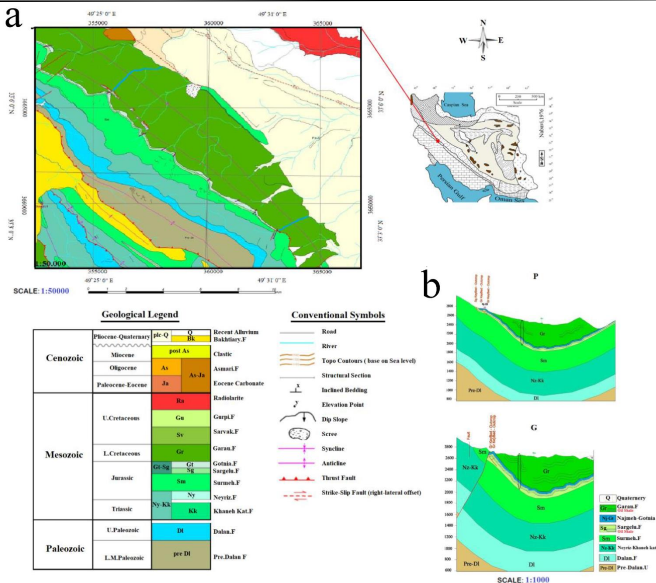
شکل ۱- ا) نقشه زمین‌شناسی (۱:۵۰,۰۰۰) منطقه، ب) جایگاه برش‌های مورد مطالعه (NIOC.exp, 2013) در منطقه
