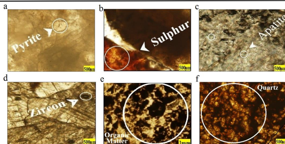
شکل ۷- تصاویر مقاطع نازک میکروسکوپی نهشته‌های مورد مطالعه: (a: پیریت، b) سولفور، c) آپاتیت، d) زیرکن، e) مواد آلی، f) دانه های کوارتز Fig. 7. Microscopic thin section images of studied deposits: a) Pyrite, b) Sulfur, c) Apatite, d) Zircon, e) Organic Matter, f) Quartz Grains
