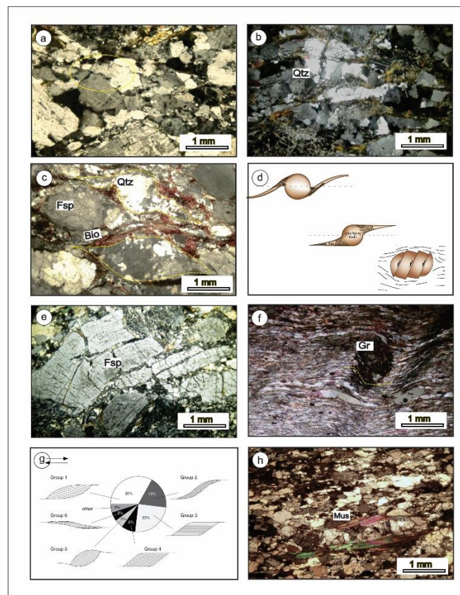
شکل ۳- تصویر میکروسکوپی ریزساختارها در میلونیت‌های زون برشی چای کور: (a) بازبلورش برآمدگی مرز دانه در کانی کوارتز (b) کوارتزهای نواری. (c) مهاجرت مرز دانه در کوارتز و پورفایروکلاست‌های سیگما و دلتا در کوارتز و فلدسپار پتاسیم (d) طبقه بندی انواع پورفایروکلاست‌ها (Fossen, 2016) (e) ساختارهای قفسه کتابی در پورفایروکلاست فلدسپار (f) پورفایروکلاست گارنت چرخیده (g) طبقه بندی انواع مینرال فیش (Ten Grotenhuis et al., 2003) (h) مسکویت فیش‌های گروه دو. همه این شاخص‌ها از مقاطع جهت دار XZ برداشت شده است که عمود بر برگواره و موازی با خطواره می‌باشد.
