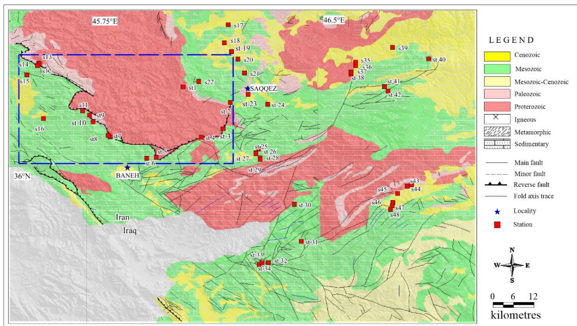
شکل ۲- نقشه زمین‌شناسی ترسیم شده محدوده سقز- بانه (Nogol-Sadat ; Alavi et al., 1976; Zahedi and Hajian, 1985; Eftekharnjad, 1973) پس از تغییر و ساده‌سازی. چهارگوش آبی رنگ محدوده راندگی اصلی منطقه سقز- بانه را نشان می‌دهد که به عنوان ساختار کلیدی در این پژوهش برگزیده شده است.
