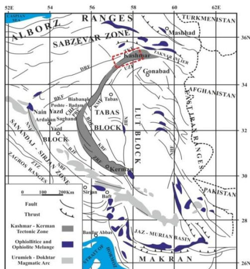
شکل ۱. موقعیت منطقه کوه‌سرهنگی در زون تکتونیکی کاشمر-کرمان پهنا ایران مرکزی [۷] به صورت چهارگوش نشان داده شده است
