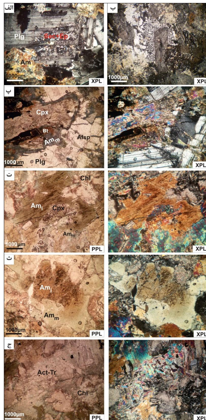
شکل ۴. تصاویر میکروسکوپی نمونه‌های گابرویی جنوب بردسکن. الف) ادخال‌های ثانوی اپیدوت و سیریسیت در بلور پلاژیوکلاز، ب) هم‌رشدی گرانوفیر در اطراف پلاژیوکلاز، پ) جای‌گزینی کلینوپیروکسن از حاشیه با آمفیبول سبز دگرگونی ( Am_m ). بخشی از این آمفیبول‌ها نیز در حال تبدیل به بیوتیت هستند، ت) بقایایی از کلینوپیروکسن بصورت ادخال در آمفیبول قهوه‌ای با منشأ ماگمایی ( Am_i )، ث) آمفیبول‌های ماگمایی قهوه‌ای از اطراف به‌وسیله آمفیبول دگرگونی حرارت کم در حال جای‌گزینی هستند، ج) اجتماعات اورالیت + کلریت که تحت شرایط دگرسانی حرارت اندک جانشین آمفیبول حرارت بیش‌تر شده‌اند
