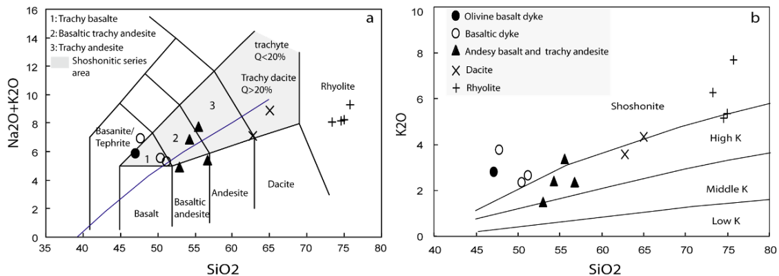
شکل ۴. (a) نمودار مجموع آلكالی‌ها در مقابل سیلیس [۱۸] و موقعیت نمونه‌ها در این نمودار، (b) نمودار K_2O در مقابل سیلیس [۱۹] و قرار گیری نمونه‌ها در محدوده کالک آلكالین و شوشونیتی
