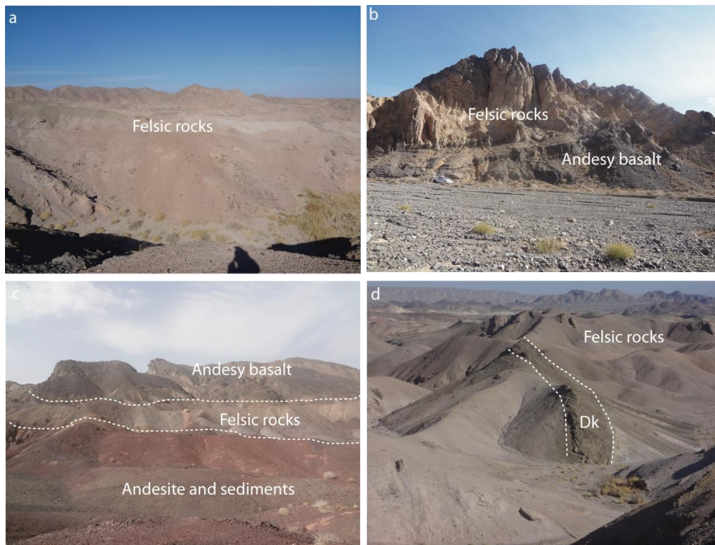
شکل ۲. روابط صحرایی واحدهای سنگی رخنمون یافته در محدوده بررسی شده، (a) رخنمون‌های گسترده سنگ‌های اسیدی در محدوده بررسی شده، (b) رخنمون سنگ‌های آندزیت بازالتی در بین سنگ‌های فلسیک، (c) توالی سنگ‌های رسوبی و آندزیتی در زیر و سنگ‌های فلسیک در بالای آن‌ها و سنگ‌های بازیک در بالاترین بخش توالی (d) دایک‌های بازالتی در بین نهشته‌های فلسیک در محدوده بررسی شده
