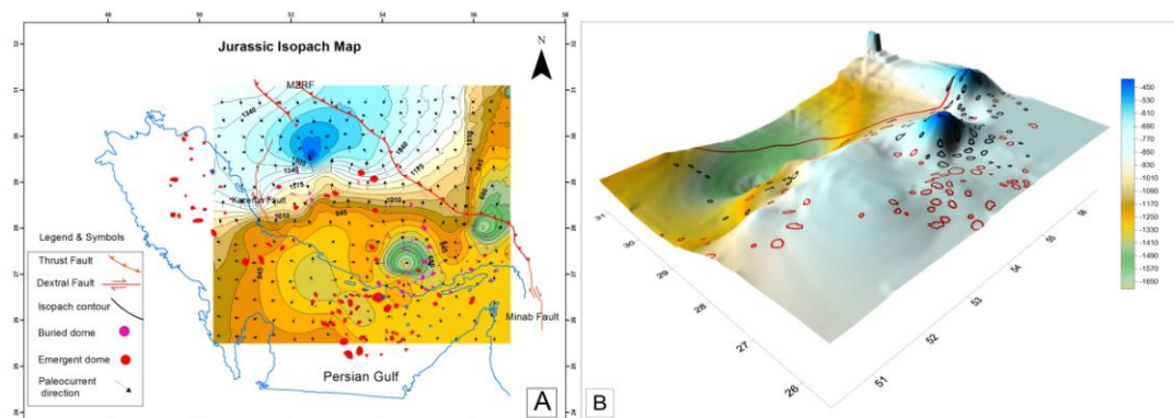
شکل ۷. A) نقشه هم‌ضخامت تهیه شده بر اساس خطوط میزان بازه زمانی ژوراسیک، B) تصویر سه‌بعدی این بازه زمانی قبل از رسوب‌گذاری
