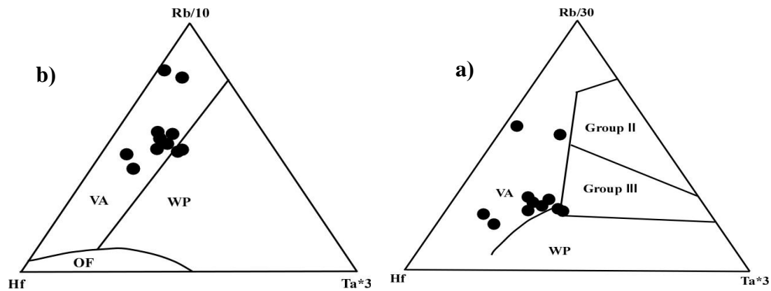
شکل ۹. نمودارهای Hf-Rb/30-Ta \times 3 و Hf-Rb/10-Ta \times 3 متمایزکننده محیط تکتونیکی گرانیتها [۷۱]. میدانهای WP: گرانیتوئیدهای درون صفحات، VA: گرانیتوئیدهای قوس آتشفشانی، OF: گرانیتوئیدهای پشته اقیانوسی و Group II: گرانیتوئیدهای همزمان با برخورد و Group III: گرانیتوئیدهای پس از برخورد را نشان می‌دهد. چنان‌که مشاهده می‌شود، نمونه‌های منطقه در محدوده قوس آتشفشانی قرار می‌گیرند
