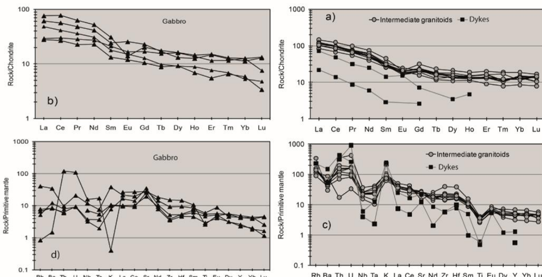
شکل ۵. نمودار عناصر نادر خاکی نرمال شده به کندریت [۳۵] و (c و d) نمودار چند عنصری نرمال شده نسبت به گوشته اولیه [۳۵]
