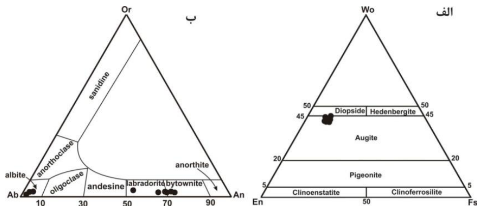
شکل ۶. الف) مطابق نمودار تقسیم‌بندی پیروکسن [۱۲]، کلینوپيروکسن نمونه‌های بررسی شده از نوع اوریت هستند، ب) با توجه به نمودار مثلثی Ab-An-Or [۱۳]، ترکیب پلاژیوکلازهای نمونه‌های گابرویی بررسی شده از نوع لابرادوریت، بیتونیت و آلپیت هستند
