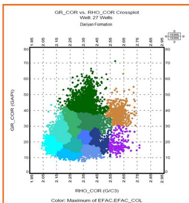
شکل ۳. ترسیم نمودار گاما مقابل چگالی. رنگ‌ها نشان‌دهنده رخساره‌های الکتریکی سازند داریان هستند
