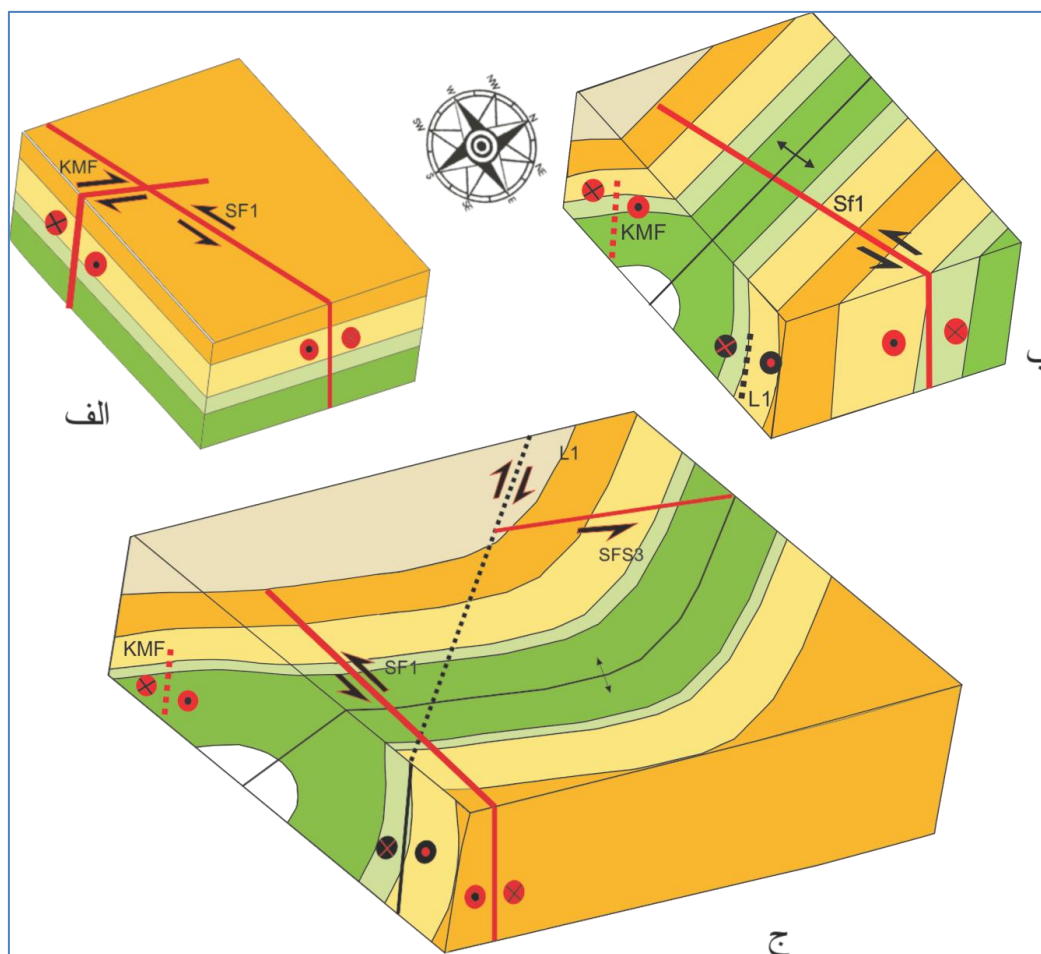
شکل ۱۵. مراحل تکامل ساختاری محدوده مطالعه الف) فعالیت گسل خارک-میش قبل از چین خوردگی و تشکیل گسل SF1، ب) تشکیل تاقدیس کوه‌های سیاه و عدم تاثیر گسل‌های عرضی بر آن، ج) فعالیت گسل L1 موجب چرخش گسل SF1 به صورت غیرفعال همراه با تاقدیس کوه‌های سیاه
