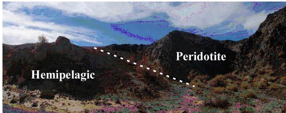
شکل ۳. نمایی از پریدوتیت‌ها در کنار رسوبات همی‌پلاژیک. مرز گسله در شکل مشخص شده است (دید به سمت جنوب)
