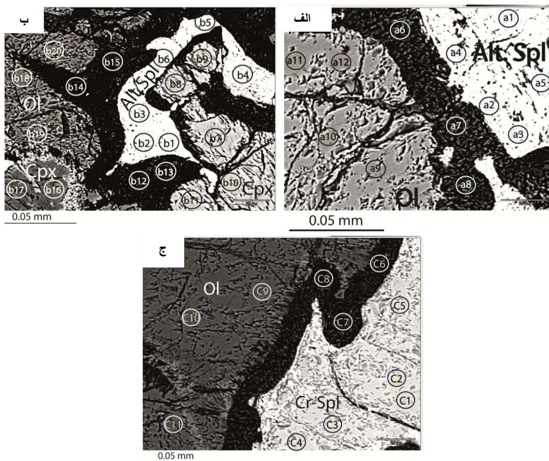
شکل ۱۰. تصاویر SEM مقطع صیقلی سنگ که محل نقاط تجزیه شده را نشان می‌دهد. داده‌ها در جدول‌های ۲ تا ۵ و شکل‌های ۱۱ و ۱۲ آمده است. الف) Alt. Spl : کروم اسپینل دگرسان، ب) Cpx : کلینوپیروکسن، Cr-Spl : کروم اسپینل سالم. ج) Ol : الیوین
