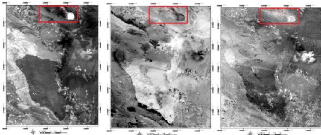
شکل ۶. چپ) نسبت باندهای ۴ به ۸ کانی‌های رسی (مناطق روشن نشان‌دهنده رس است)، وسط) تصویر تحلیل مؤلفه اصلی مقدار منفی در باند ۴ (مناطق تیره نشان‌دهنده رس است)، راست) تصویر کم‌ترین مربعات با باند مدل ۴ (مناطق روشن نشان‌دهنده رس است)
