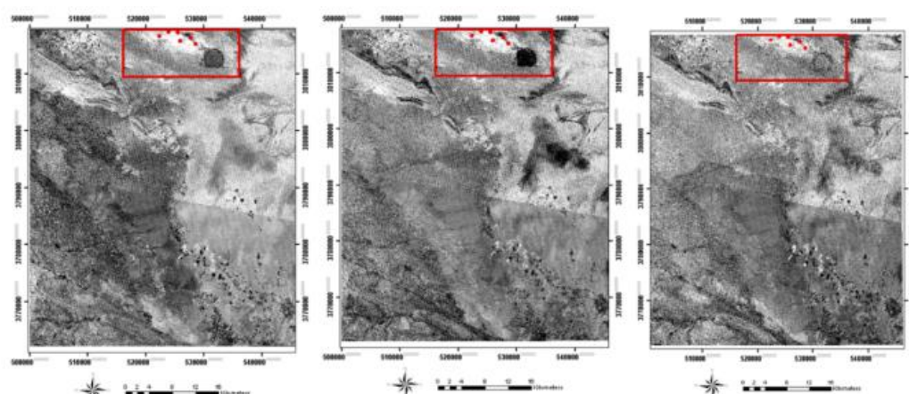
شکل ۷. چپ) تصویر نسبت باندهای ۲ به ۱ (مناطق روشن بسترهای غنی آهن است)، وسط) تصویر کروستا با باندهای ۱-۲-۳-۴ با مقدار مؤلفه اصلی در باند ۴ (مناطق روشن بسترهای غنی آهن است)، راست) تصویر روش کم‌ترین مربعات با باند مدل ۲ (مناطق روشن بسترهای غنی آهن است).
