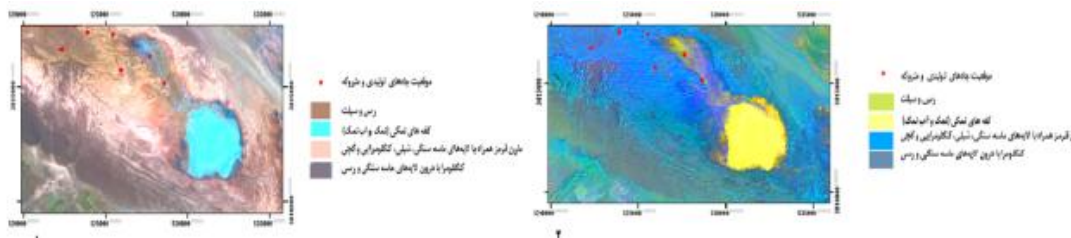
شکل ۱۰: تصویر مرکب منطقه بررسی شده، (۱) (۴/۸-۳/۴-۲/۱) ، (۲) (۴/۸-۳/۴-۲/۱) .
