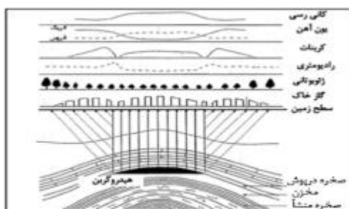
شکل ۱. نمود و تراوش هیدروکربنی در سطح [۷]
