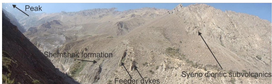
شکل ۲. نمایی از دره گزنه و واحدهای تشکیل دهنده دیواره شمالی
