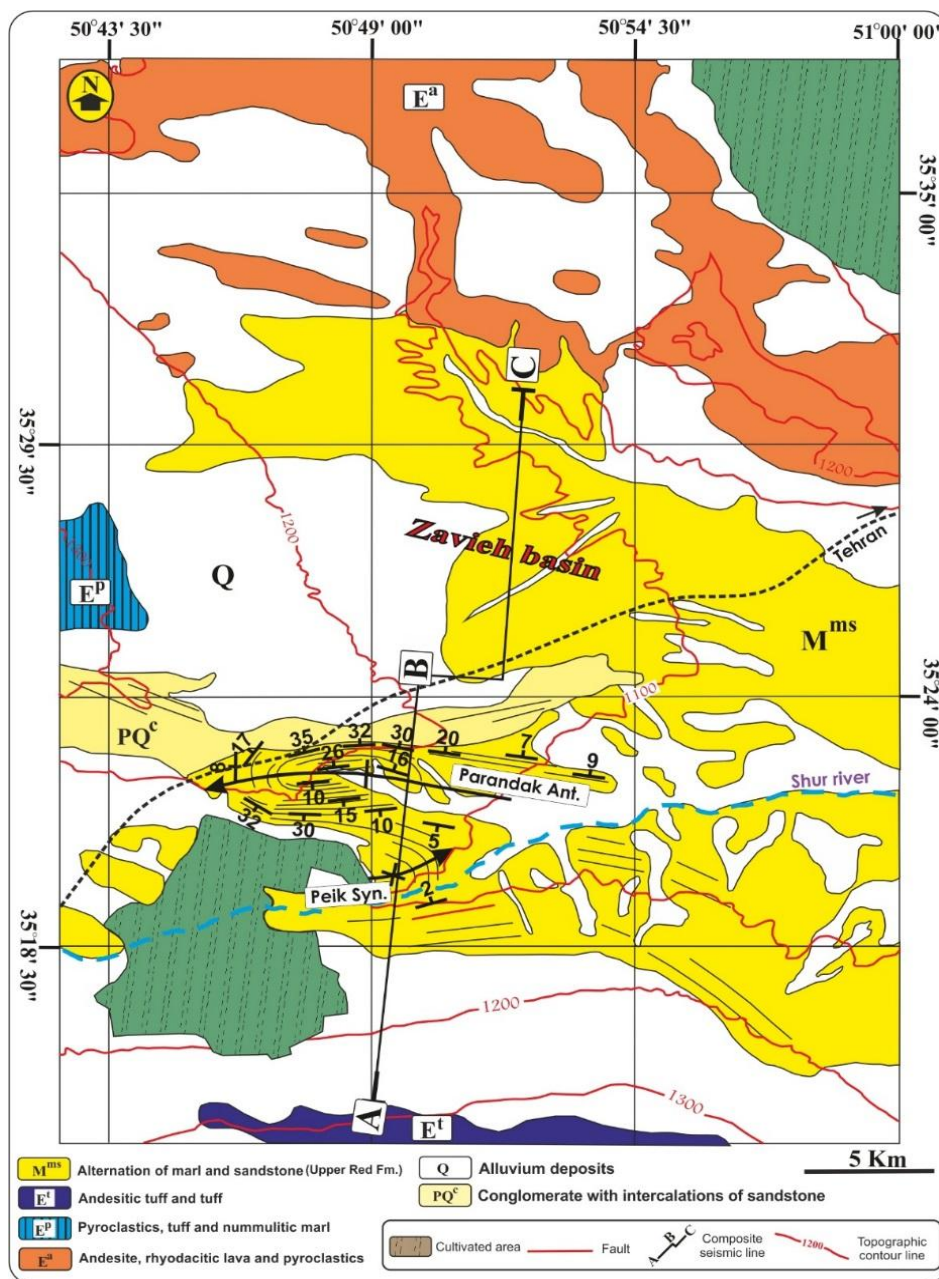
شکل ۳. نقشه زمین‌شناسی از بخش شمال غربی حوضه زاویه (تهیه شده بر اساس مشاهدات صحرایی و تصاویر ماهواره‌ای). محل گذر خط لرزه‌ای ترکیبی ABC در شکل نشان داده شده است. چین خوردگی‌های امین‌آباد و پرندک دو تاق‌دیس اصلی توسعه یافته در این حوضه رسوبی به‌شمار می‌آیند.
