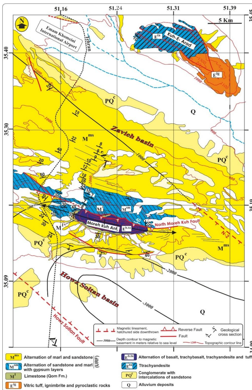
شکل ۶. نقشه زمین‌شناسی از بخش شمالی حوضه‌های زاویه و حوض سلطان، تهیه شده بر اساس تصاویر ماهواره‌ای، مشاهدات صحرائی، نقشه مغناطیس هوایی تهران [۱۶] و داده‌های منتشر شده در برگه زمین‌شناسی رباط کریم با مقیاس ۱:۱۰۰۰۰۰ [۴]. محل مقطع ساختمانی AA' (شکل ۷ آ) در نقشه مشخص شده است.
