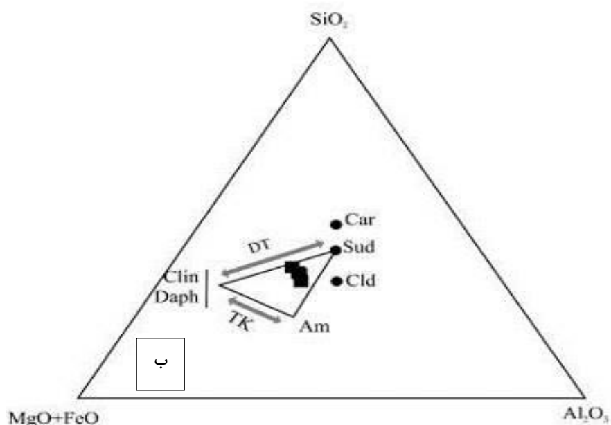
شکل ۸. آ) ترکیب شیمیایی میکای سفید روی نمودار MgO+FeO, Al_2O_3, K_2O [۲۱]. دایره توپر نشان‌گر میکای سفید موجود در مرکز بلاست‌های پلاژیوکلاز. مربع توپر نشان‌گر مرکز میکای سفید موجود در شیبستوزیته اصلی. دایره توخالی نشان‌گر حاشیه میکای سفید موجود در شیبستوزیته اصلی، ب) ترکیب شیمیایی کلریت روی نمودار SiO_2, MgO+FeO, Al_2O_3 [۲۱]
