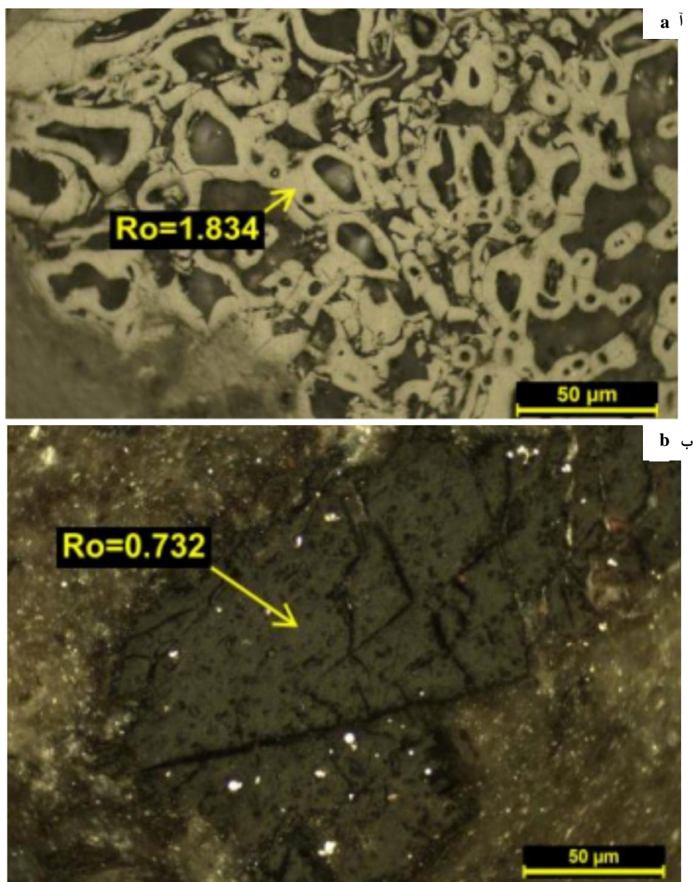
شکل ۴. تصاویر میکروسکوپی نور بازتابی از ماسرال‌های با درصد بازتاب ویتترینیت در (آ) نمونه زغال سنگ درجه بالا (نمونه K19T5) و (ب) نمونه زغال سنگ درجه پایین (K8T3) از معدن تخت Figure 4. Reflected light microscopic images of macerals with different vitrinite reflectance percentages in (a) high-grade coal sample (K19T5 sample) and (b) low-grade coal sample (K8T3) from the Takht mine.
