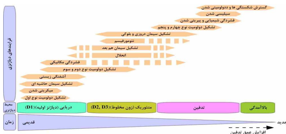
شکل ۱۶. توالی پاراژنز سازند الیکا در مناطق بررسی شده
