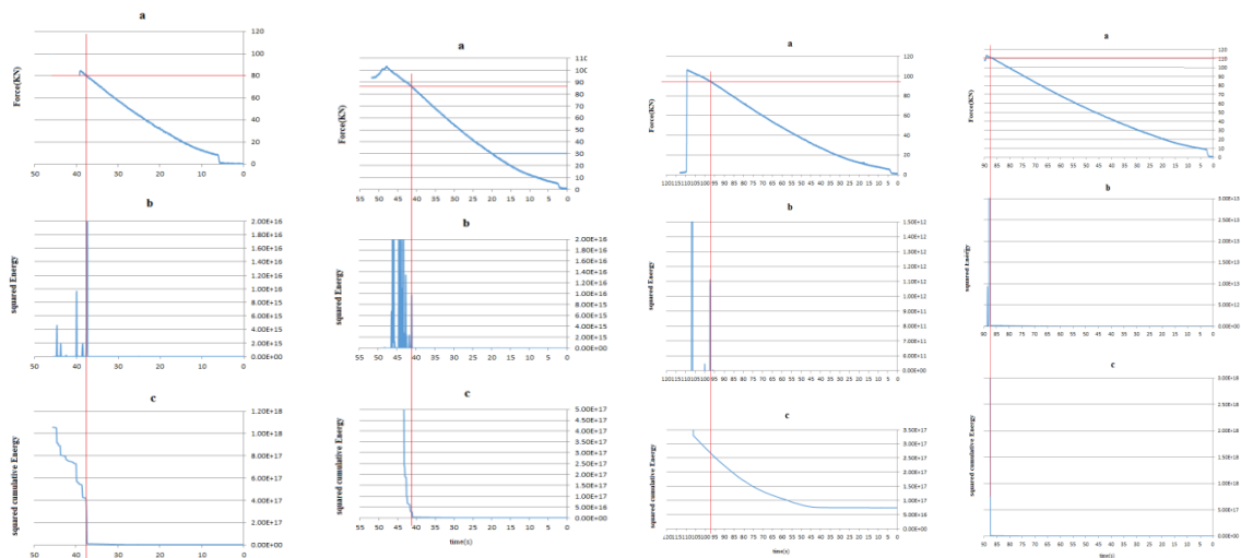
شکل ۱۰. نمودار بارگذاری، انرژی و انرژی تجمعی بر حسب زمان برای نمونه sc1-60
