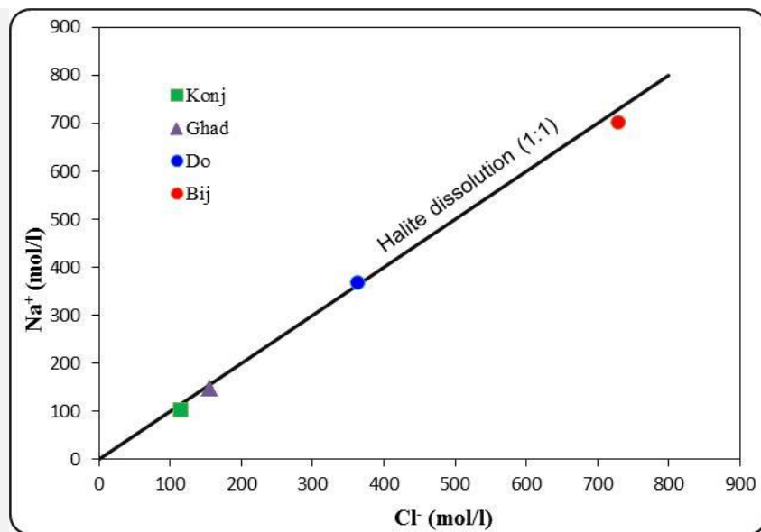
شکل ۸. نمودار رابطه Na به Cl چشمه‌های گوگردی تنگ بیجار، قدح، کنجانچم و دویرج Fig. 8. Na/Cl diagram of Tang Bijar, Ghedah, Konjancham and Doiraj sulfur springs.
