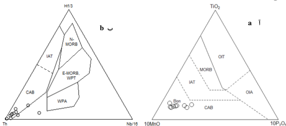
شکل ۹. نمودارهای تعیین محیط تکتونیکی، که سنگ‌های گابرویی کوه ارغون روی آنها ترسیم شده‌اند. (آ) نمودار TiO_2-10*MnO-10*P_2O_5 (Mullen, 1983). (ب) نمودار Th-Hf/3-Nb/16 (Wood, 1980). Figure 9. Tectonomagmatic discriminant diagrams for the gabbroic rocks of Arghun Mountain, a) TiO_2-10*MnO-10*P_2O_5 diagram (Mullen, 1983), b) Th-Hf/3-Nb/16 diagram (Wood, 1980).
